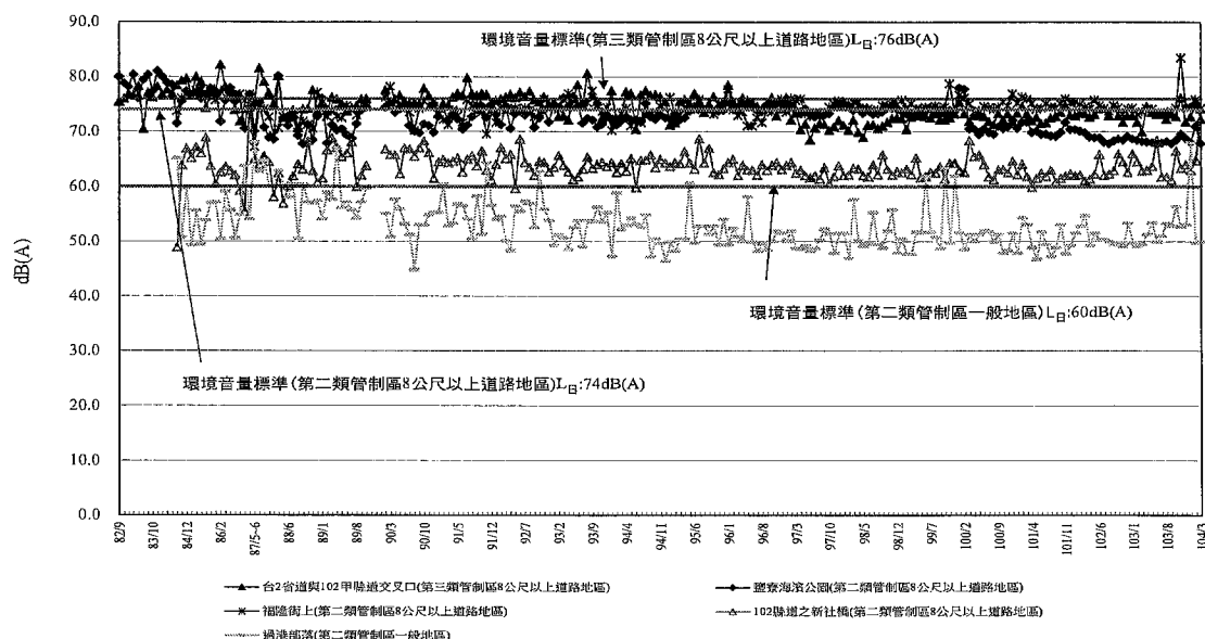
核四施工環境監測歷年噪音 L_B 非假日監測結果變化圖
