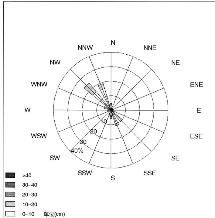
圖2.15-3 核四施工期間環境監測104年第1季 海流儀實測流速流向玫瑰圖
