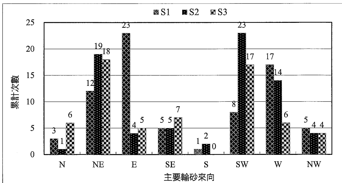
圖 3.1-43 各測站主要輸砂來向歷年累計次數比較圖
