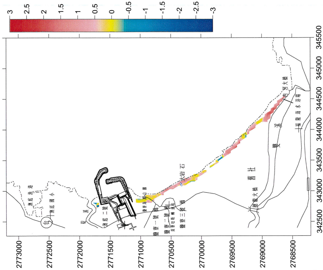
圖3.1-57 核四施工期間環境監測海岸地形 104年3月與94年11月（海事工程完工後） 侵淤比較圖
