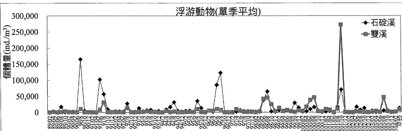
圖3.1-30 核四施工期間環境監測河域生態長期趨勢分析
