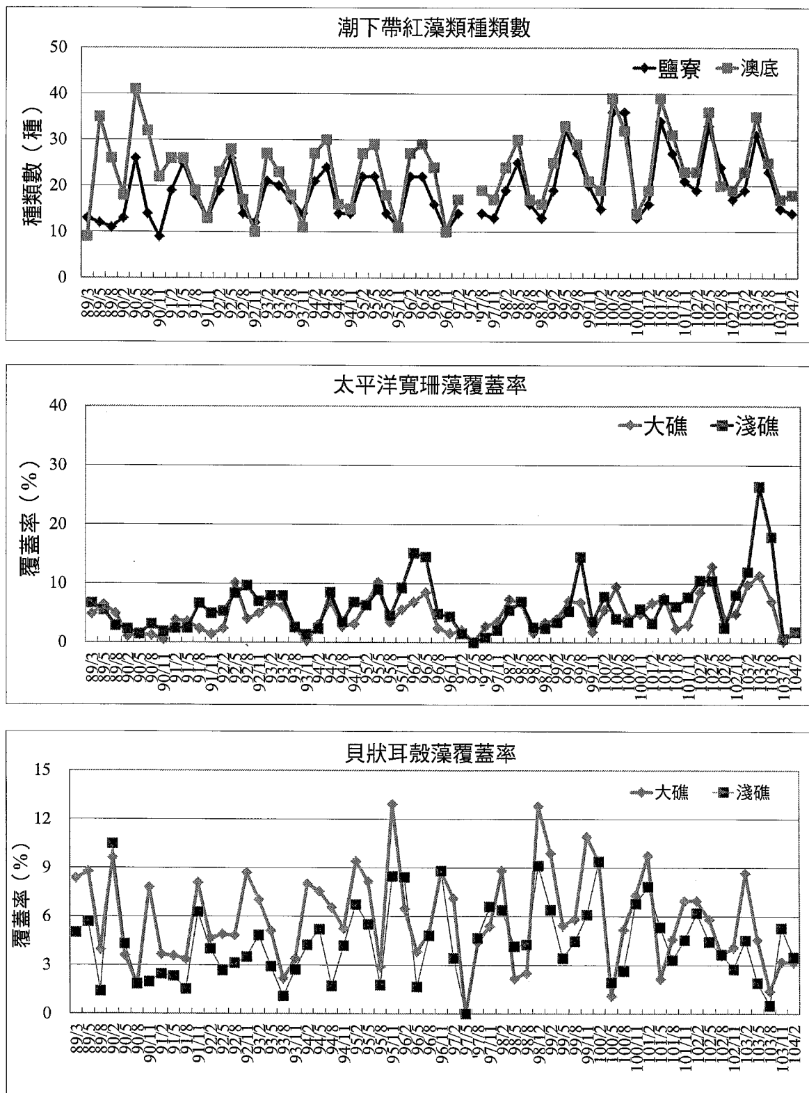
圖3.1-39 核四施工期間環境監測調查海域大型藻類指標物種長期變動趨勢
