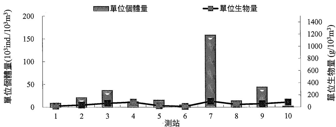
圖2.11-2 核四廠附近海域浮游動物104年第1季 各監測站個體量與生物量垂直分佈
