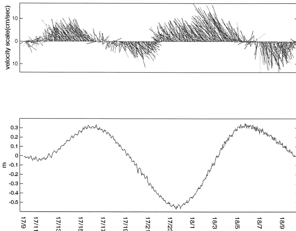
圖2.15-4 核四施工期間環境監測104年第1季流速流向 棍棒圖及潮汐水位變化圖
