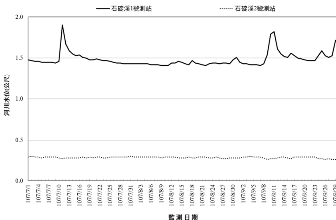
圖 2.2-1 核四封存期間河川水文 107 年 7~9 月水位變化圖
