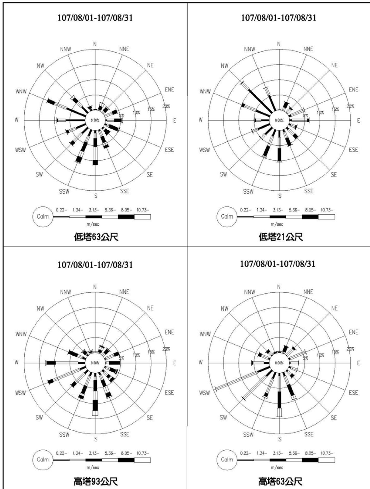
圖 2.1-2 核四封存期間環境監測氣象塔 107 年 8 月風花圖
