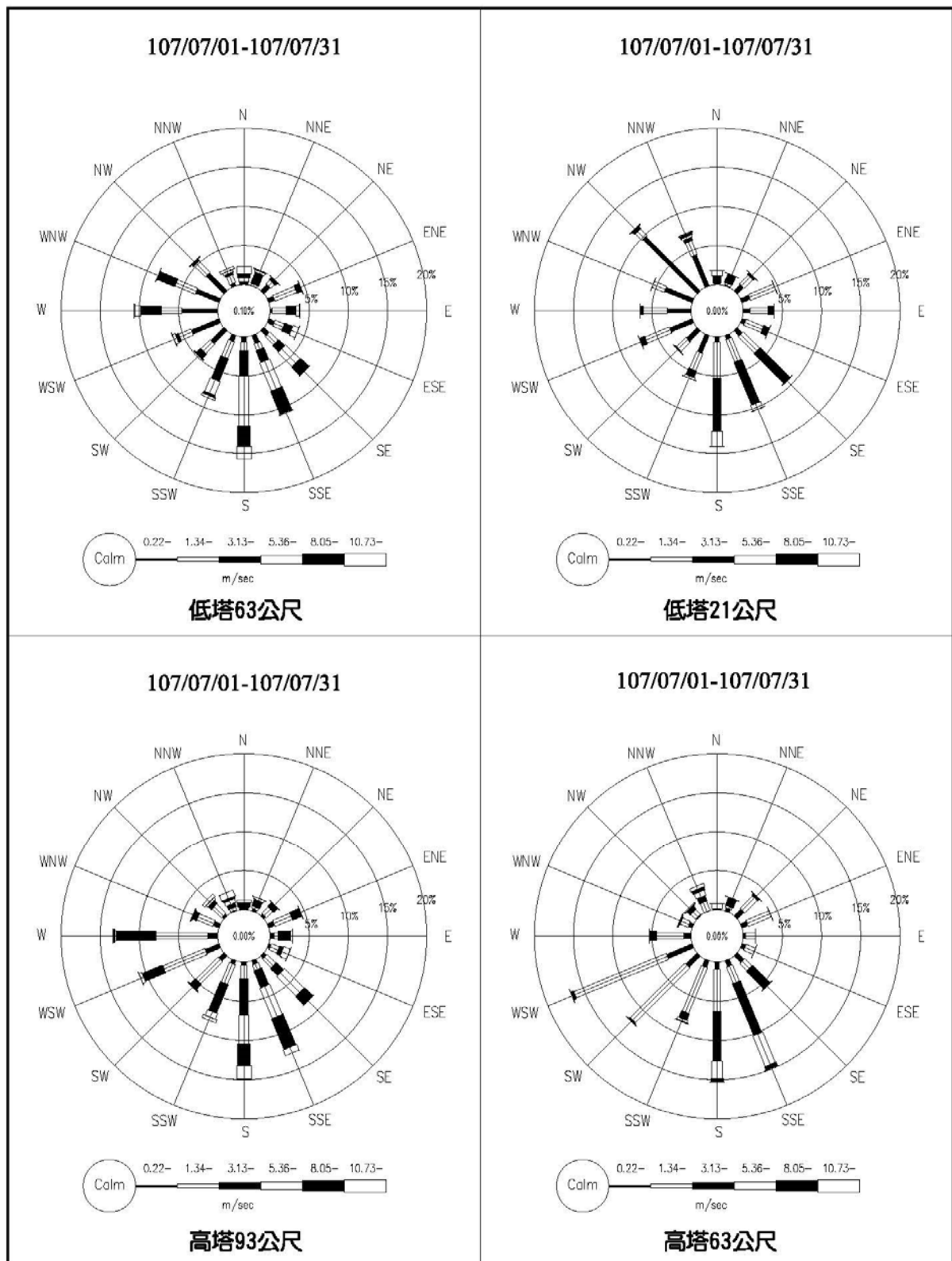
圖 2.1-1 核四封存期間環境監測氣象塔 107 年 7 月風花圖
