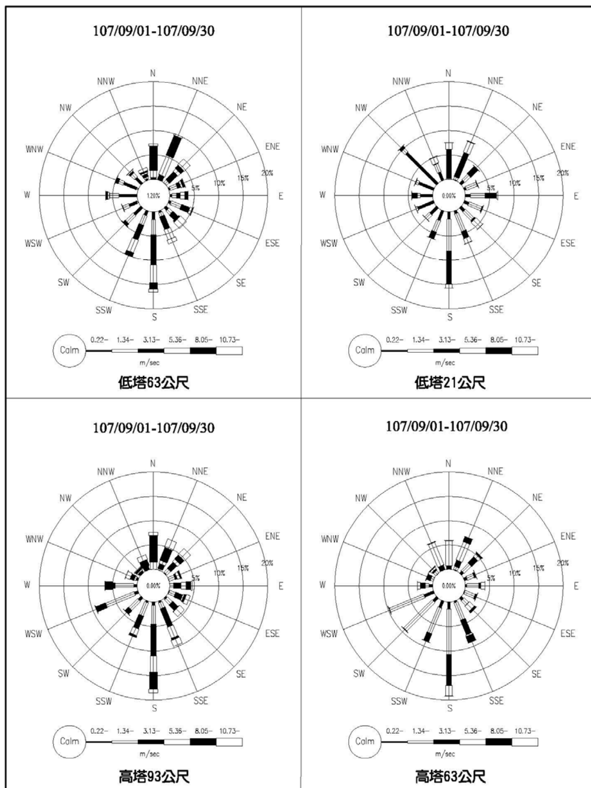
圖 2.1-3 核四封存期間環境監測氣象塔 107 年 9 月風花圖
