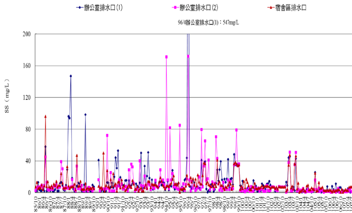
圖 3.1-8 核四環境監測廠區水質歷年調查懸浮固體濃度變化圖
