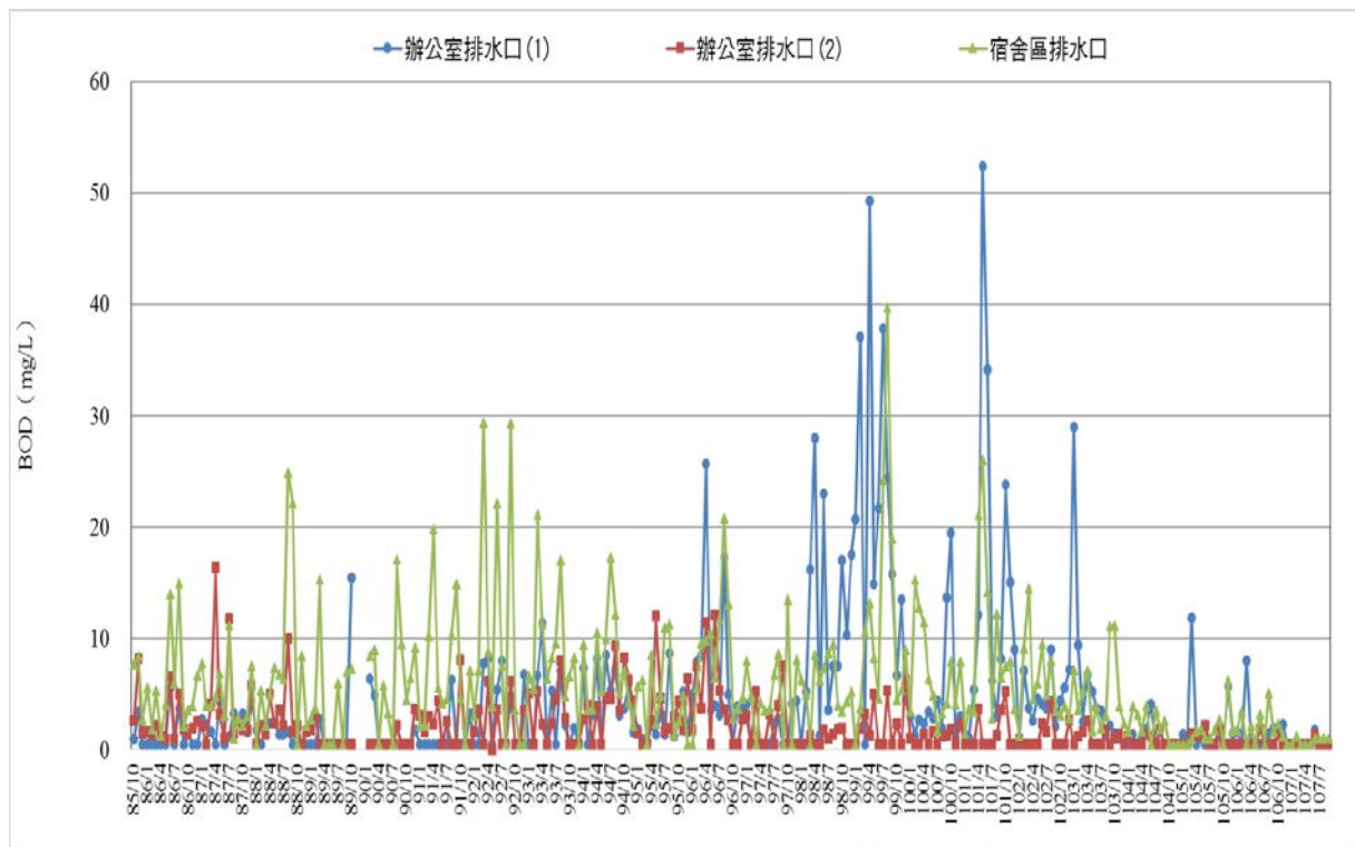
圖 3.1-9 核四環境監測廠區水質歷年調查生化需氧量變化圖
