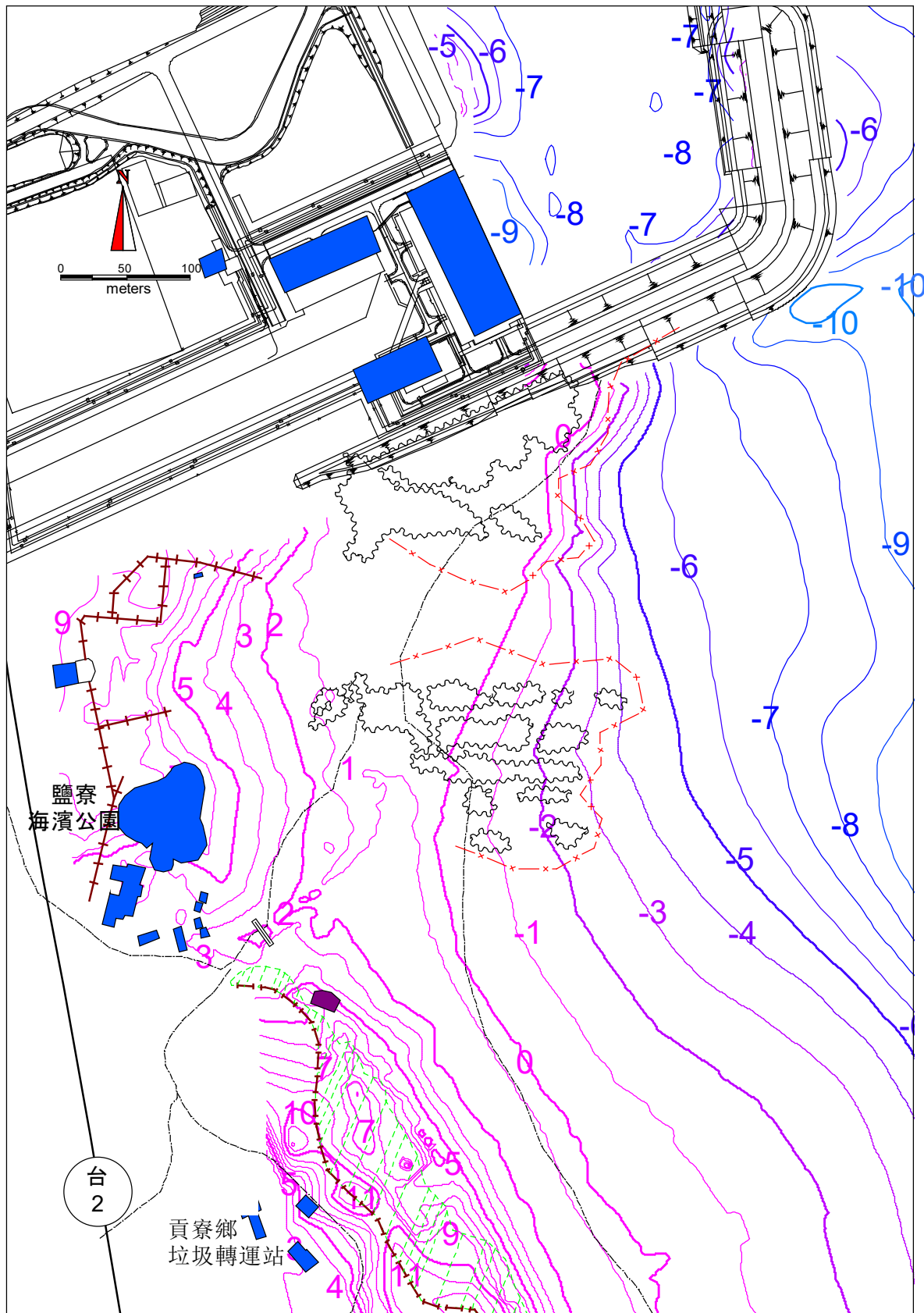
圖 2.5-3 核四封存期間鹽寮公園附近 111 年第 2 季 海岸地形監測結果
