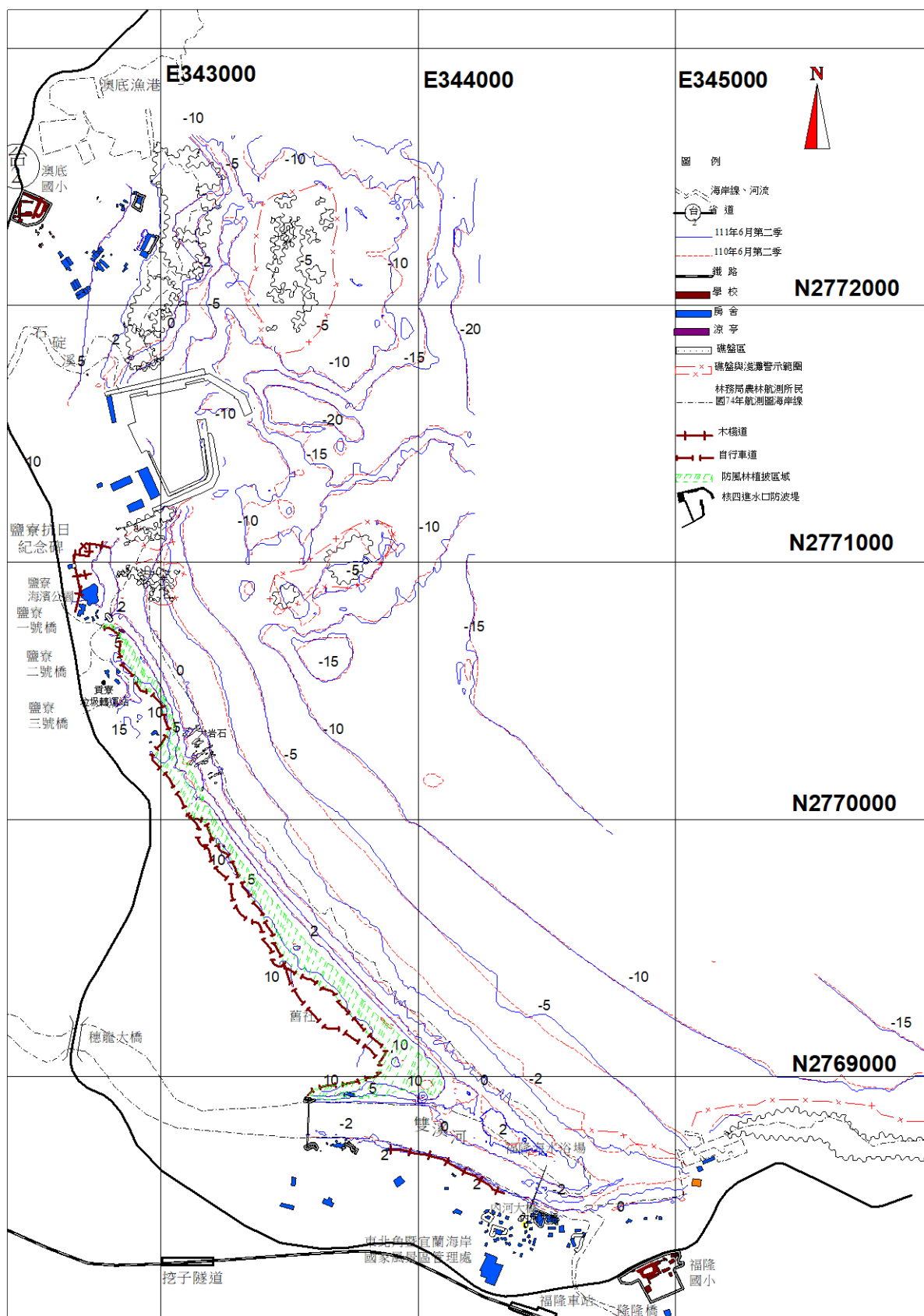
圖 3.1-10 核四環境監測海岸地形 111 年 6 月與 110 年 6 月 監測結果比較
