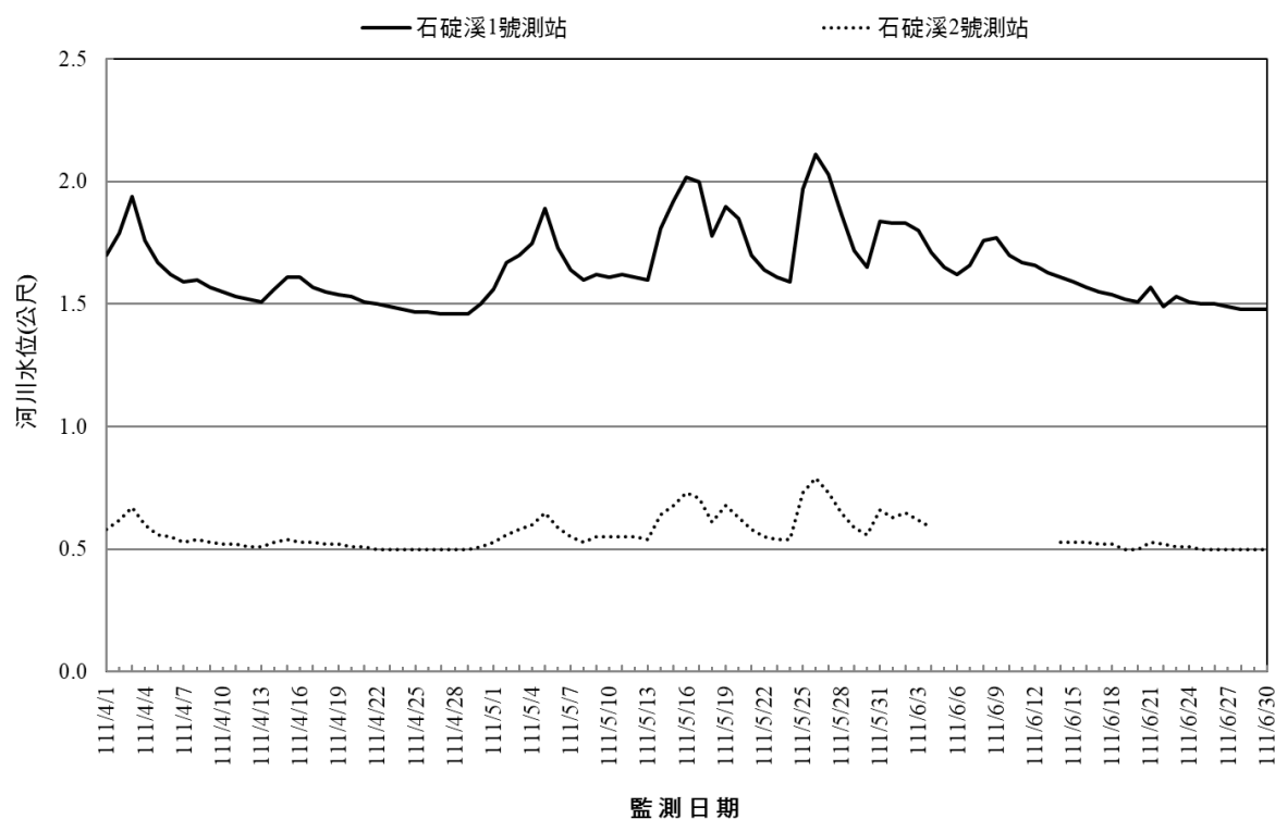
圖 2.2-1 核四封存期間河川水文 111 年 4~6 月水位變化圖
