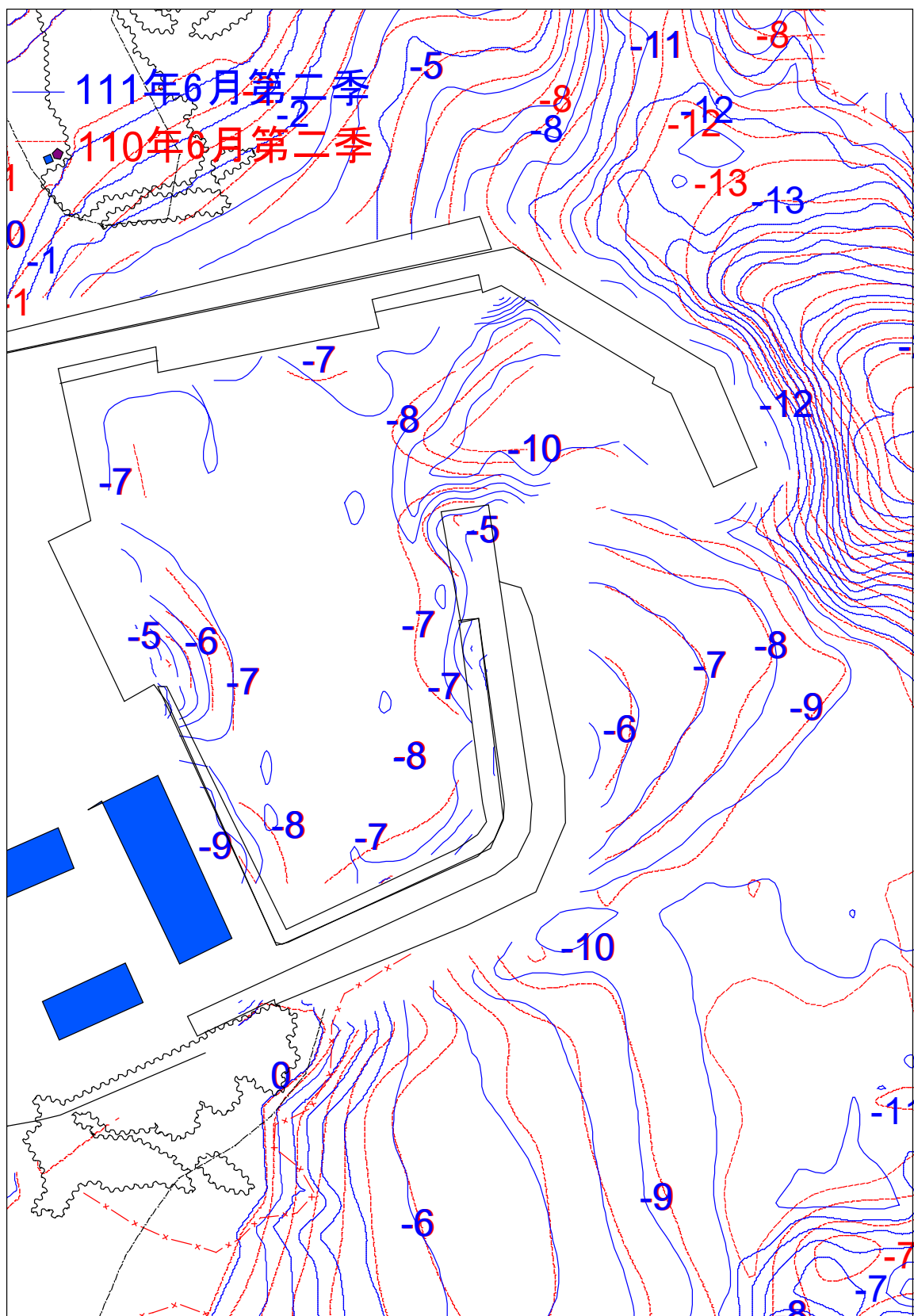
圖 3.1-11 核四環境監測海岸地形進水口防坡堤 111 年 6 月與 110 年 6 月監測結果比較
