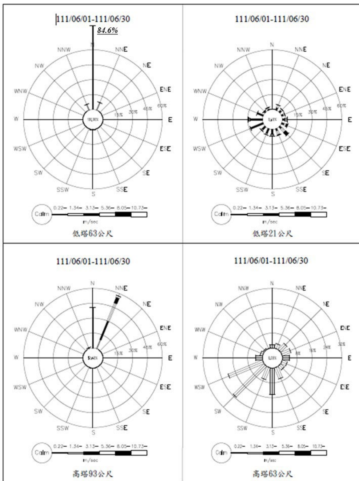
圖 2.1-3 核四封存期間環境監測氣象塔 111 年 6 月風花圖
