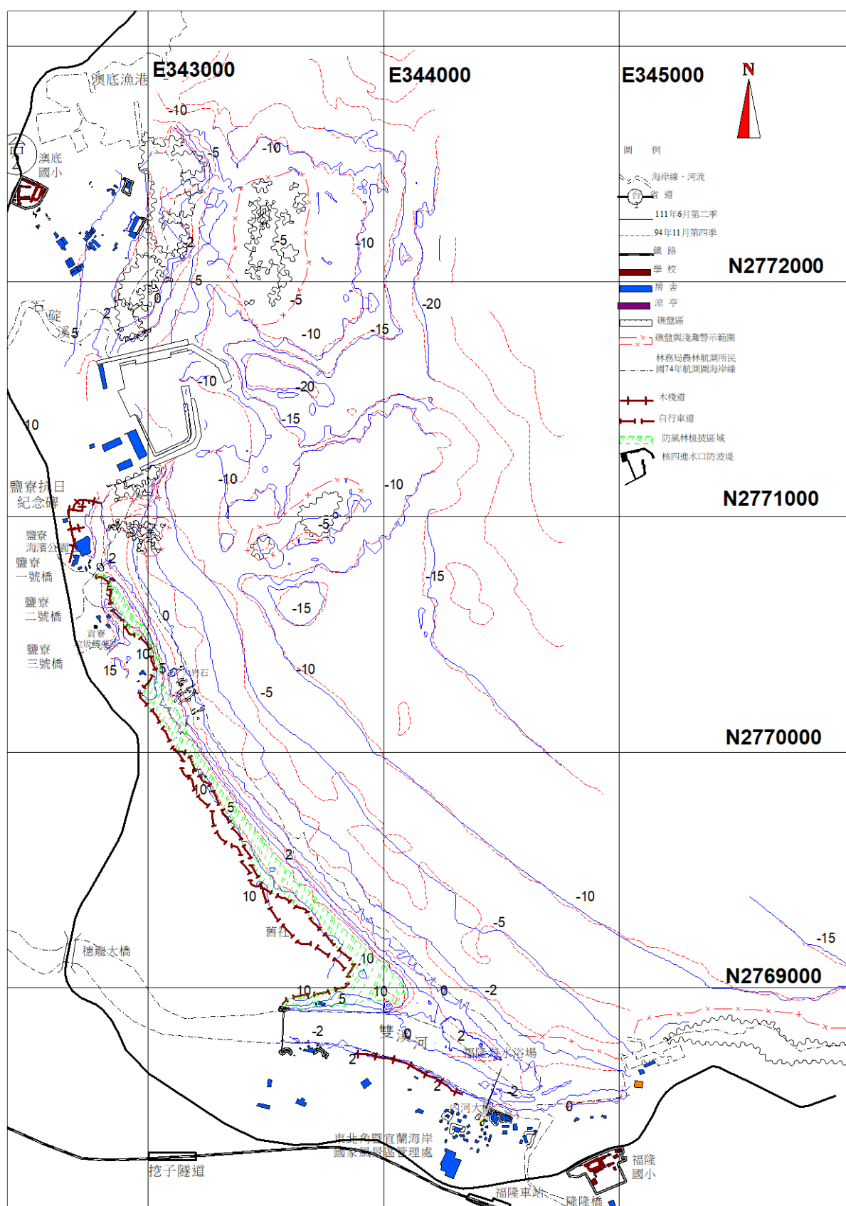
圖 3.1-14 核四環境監測海岸地形 111 年 6 月與 94 年 11 月（海事工程完工後）監測結果比較
