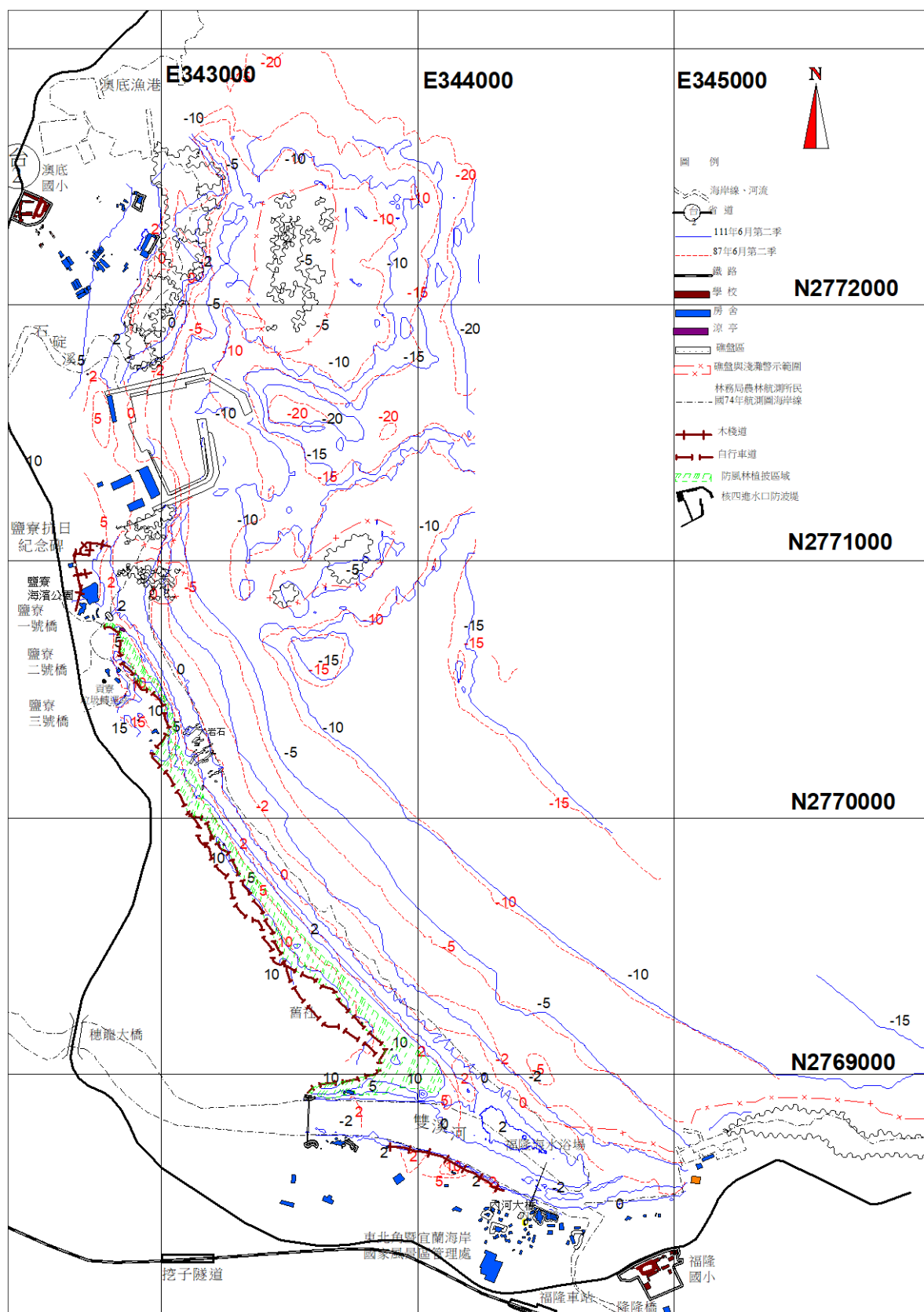
圖 3.1-13 核四環境監測海岸地形 111 年 6 月與 87 年 6 月（海事工程施工前）監測結果比較
