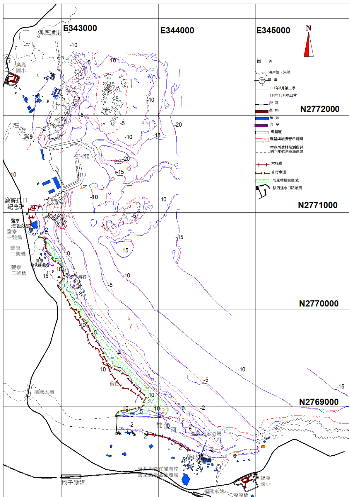
圖 2.5-5 核四封存期間海岸地形 111 年第 2 季與 110 年第 4 季監測結果比較
