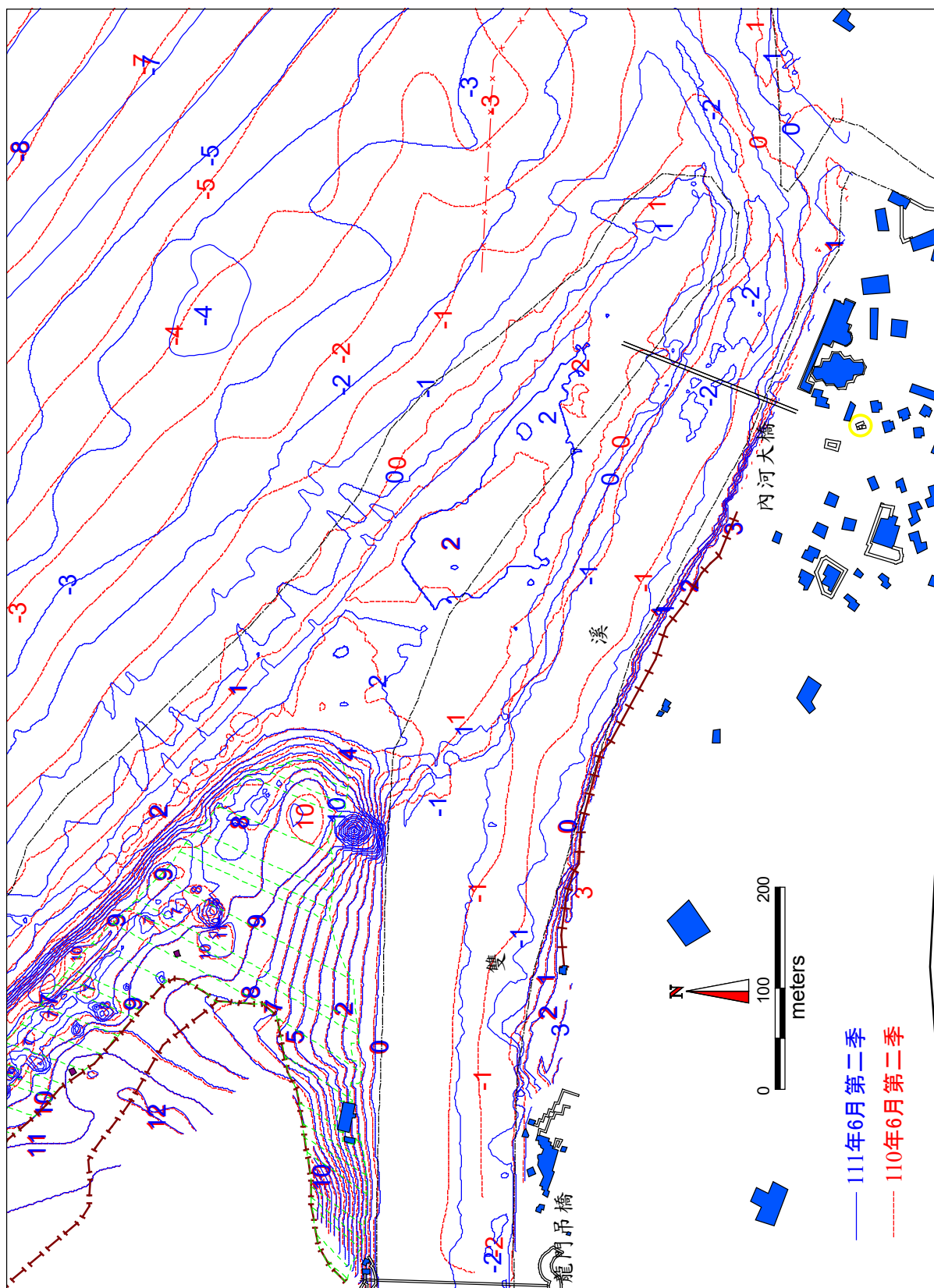
圖 3.1-12 核四環境監測海岸地形福隆附近 111 年 6 月與 110 年 6 月監測結果比較
