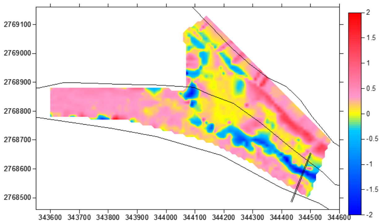
(A)111 年第 2 季與 110 年第 4 季福隆海水浴場侵淤比較圖
