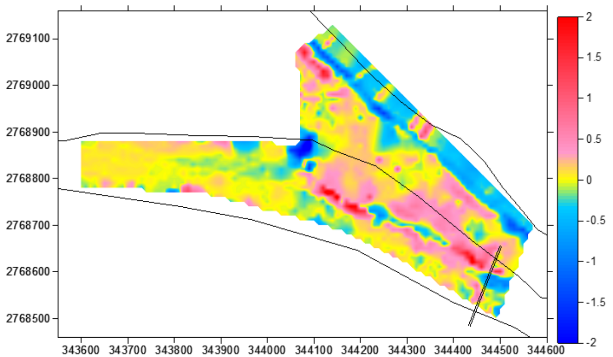
(B)111 年第 2 季與 110 年第 2 季福隆海水浴場侵淤比較圖
