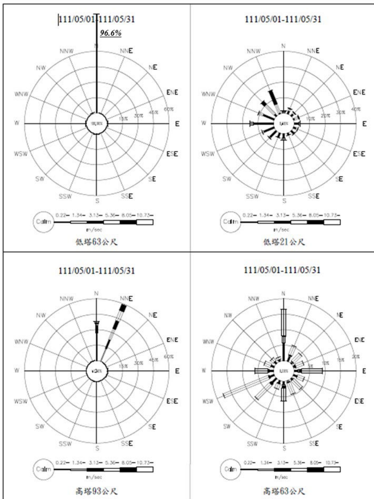
圖 2.1-2 核四封存期間環境監測氣象塔 111 年 5 月風花圖
