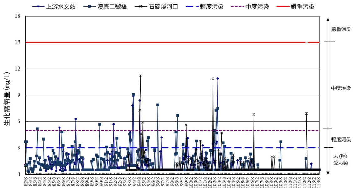
核四封存期間環境監測歷年河川水質之生化需氧量監測結果變化圖
