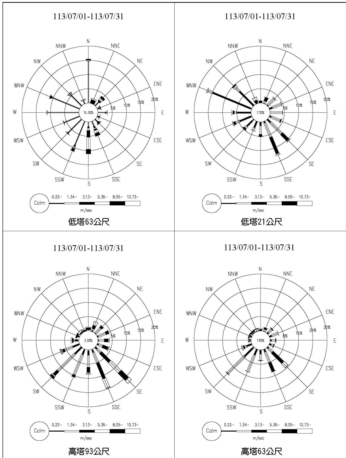
圖 2.1-1 核四封存期間環境監測氣象塔 113 年 7 月風花圖
