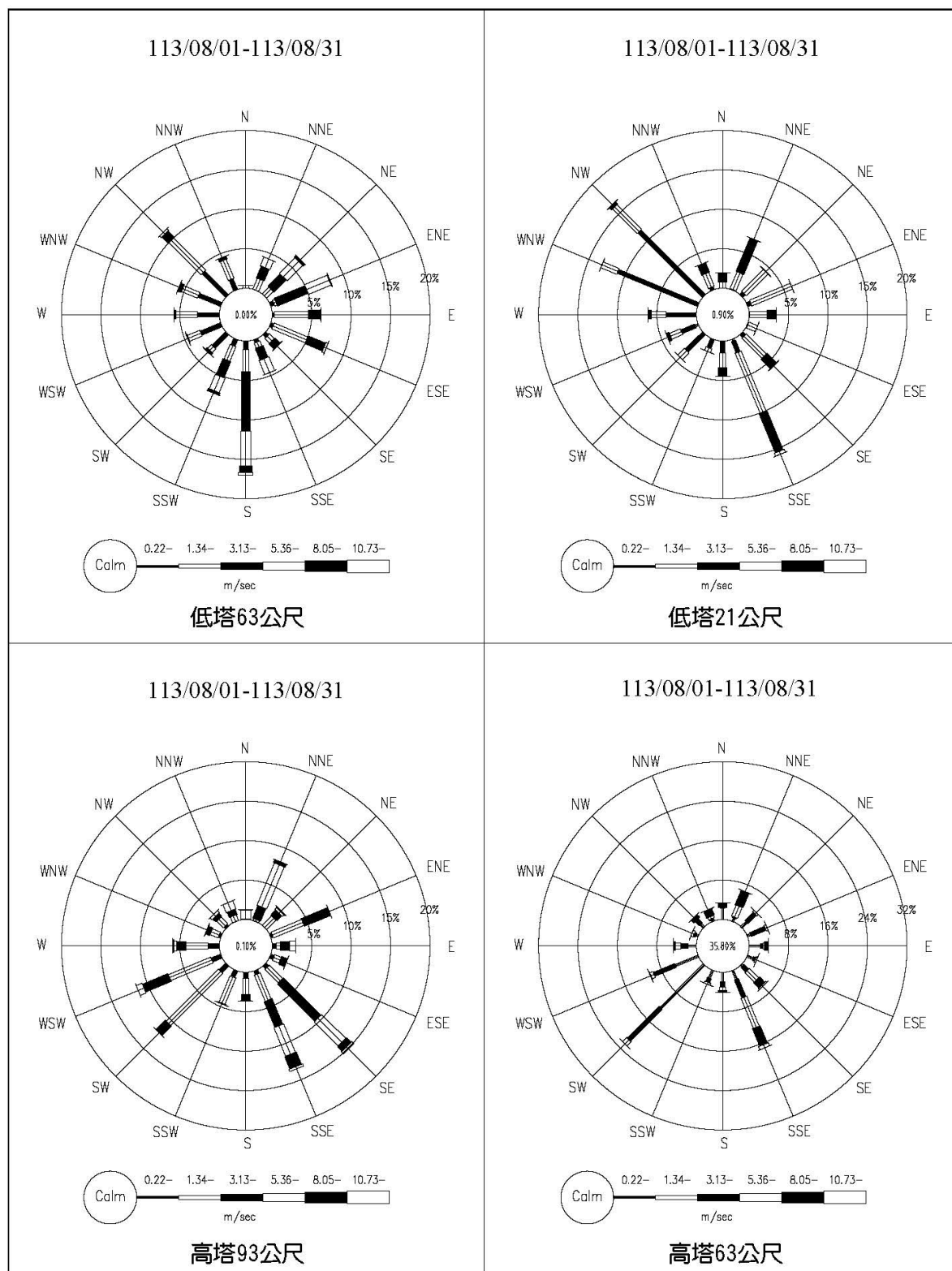
圖 2.1-2 核四封存期間環境監測氣象塔 113 年 8 月風花圖
