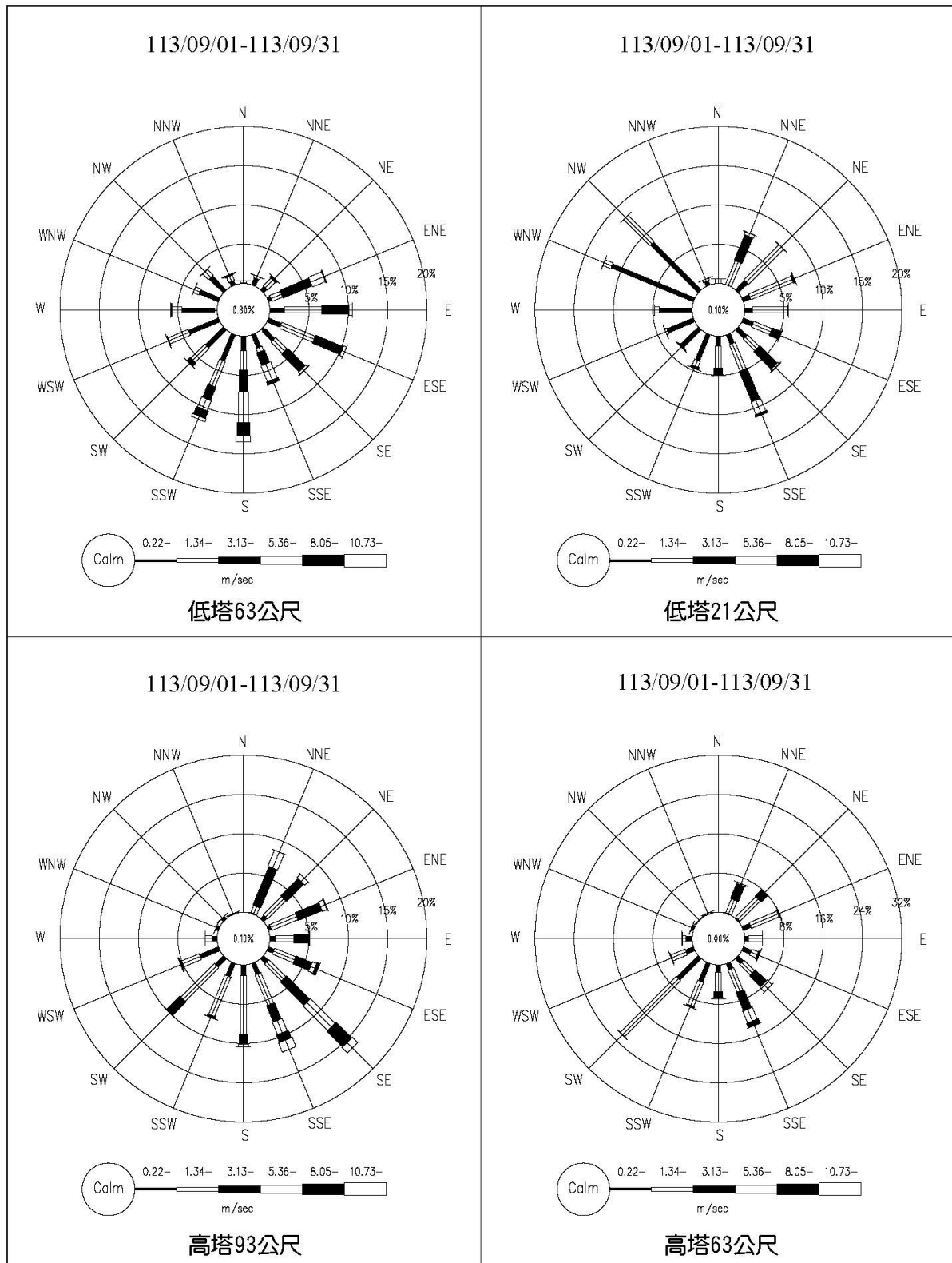
圖 2.1-3 核四封存期間環境監測氣象塔 113 年 9 月風花圖
