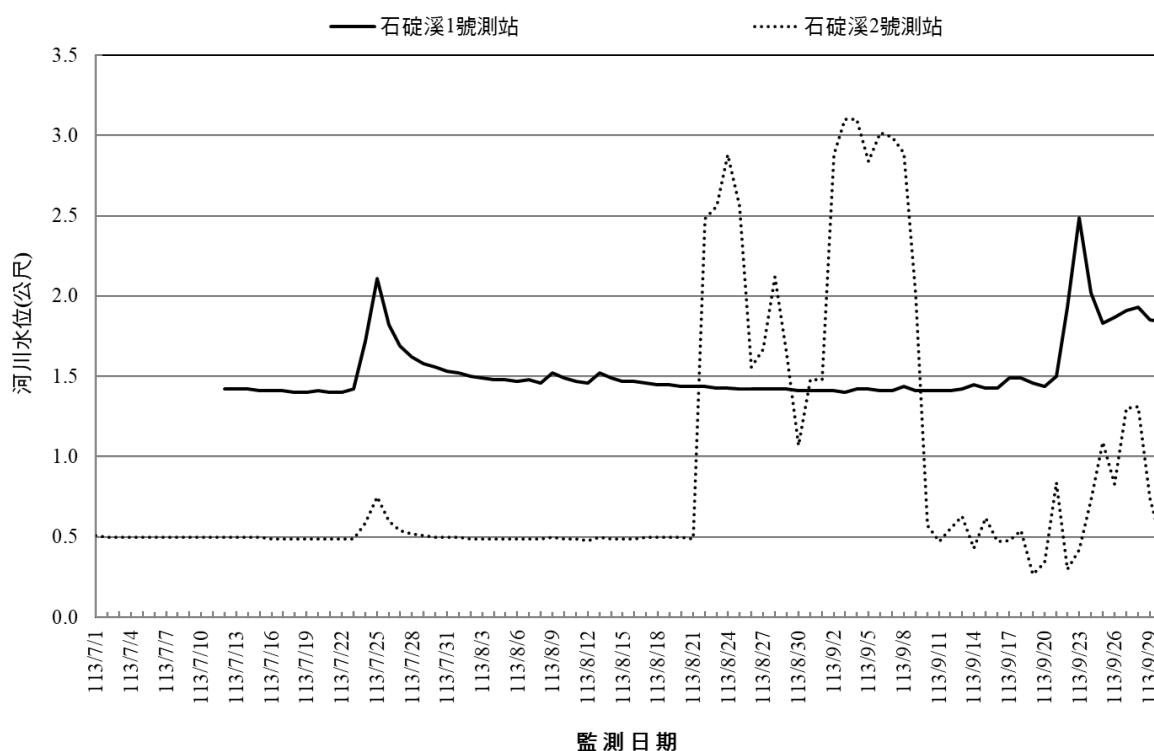
圖 2.2-1 核四封存期間河川水文 113 年 7~9 月水位變化圖
