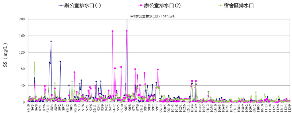
核四封存期間環境監測歷年廠區水質懸浮固體監測結果變化圖
