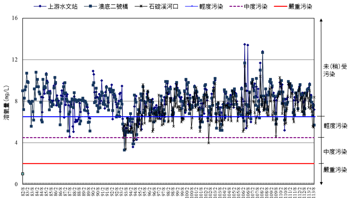
圖 3.1-2 核四環境監測河川水質歷年調查溶氧量變化圖
