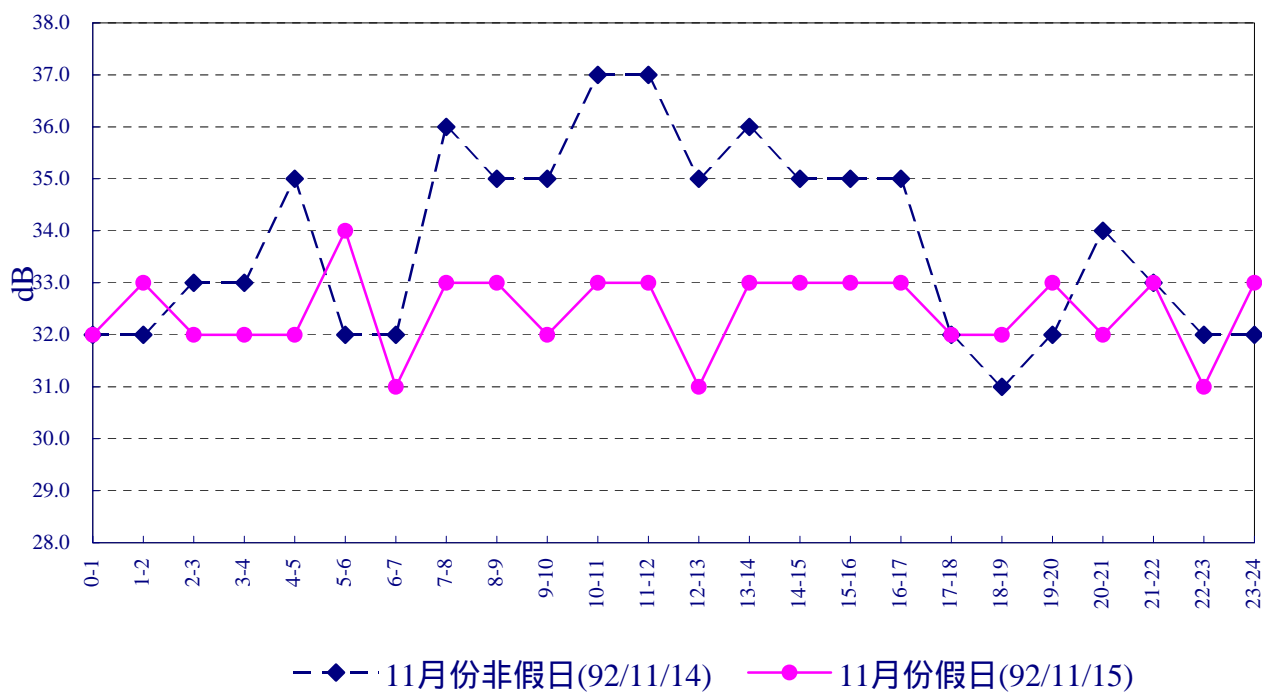
圖2.3-14 核四施工環境監測鹽寮海濱公園 92年11月振動 L_{v10} 逐時變化圖
