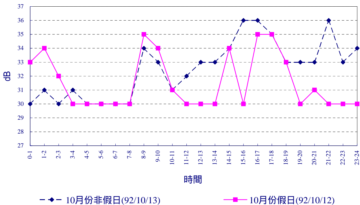
圖2.3-8 核四施工環境監測 102縣道之新社橋92年10月振動Lv 10 逐時變化圖
