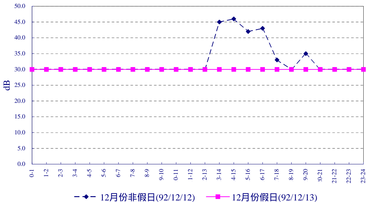
圖2.3-30 核四施工環境監測過港部落92年12月振動 L_{v10} 逐時變化圖
