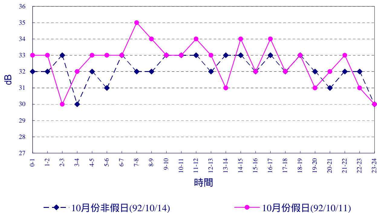
圖2.3-4 核四施工環境監測鹽寮海濱公園 92年10月振動Lv 10 逐時變化圖
