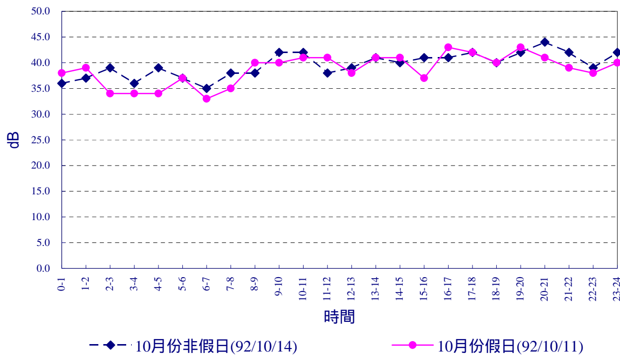
圖2.3-2 核四施工環境監測台 2與縣102甲交叉口92年10月振動 L_{v_{10}} 逐時變化圖
