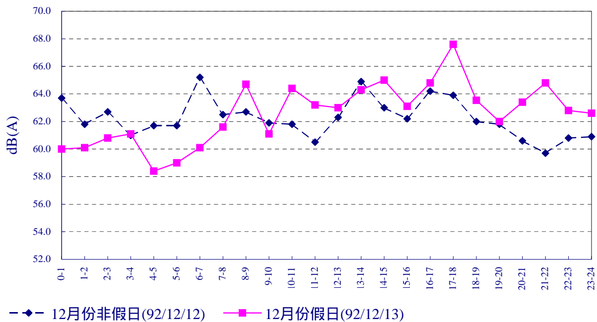
圖2.3-27 核四施工環境監測102縣道之新社橋92年12月噪音 L_{eq} 逐時變化圖
