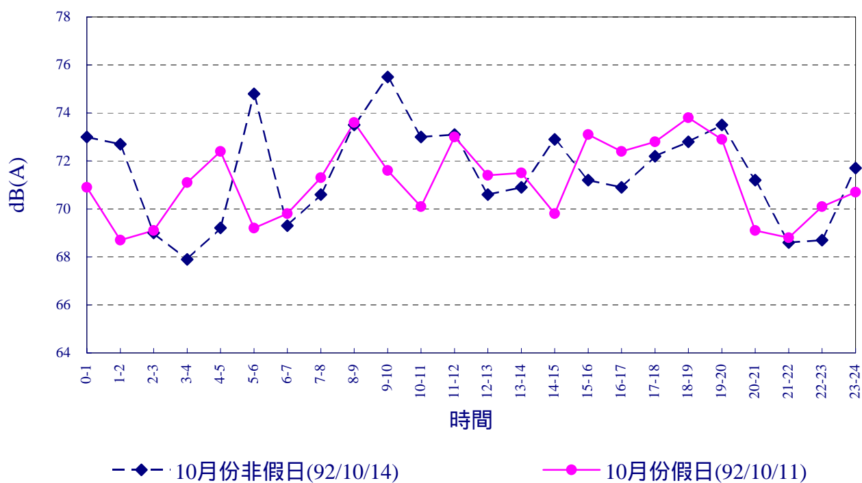
圖2.3-3 核四施工環境監測鹽寮海濱公園 92年10月噪音Leq逐時變化圖
