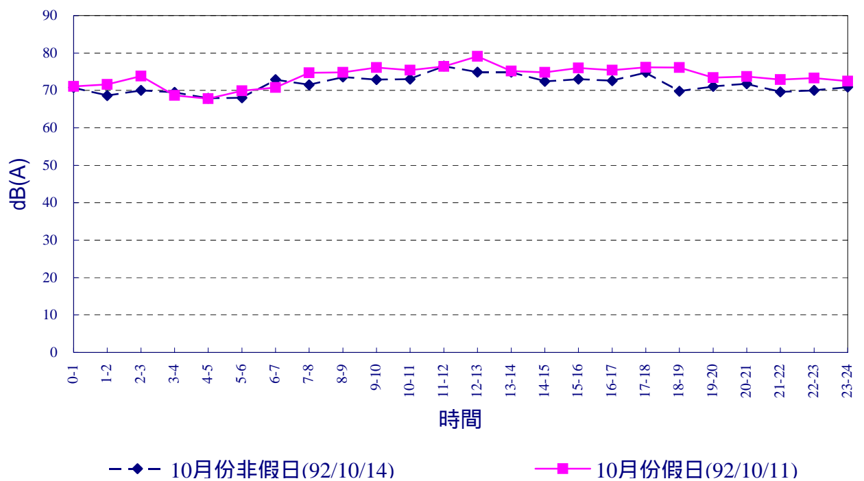
圖2.3-5 核四施工環境監測福隆街上 92年10月噪音 L_{eq} 逐時變化圖
