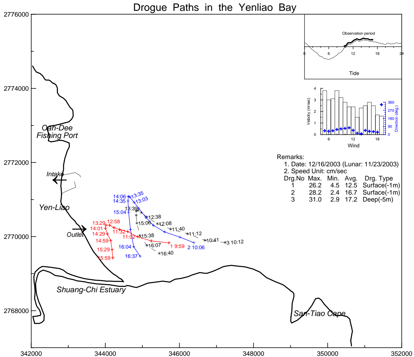
圖2.13-3 核四施工環境監測海象調查92年12月16日漂流浮標追蹤軌跡圖
