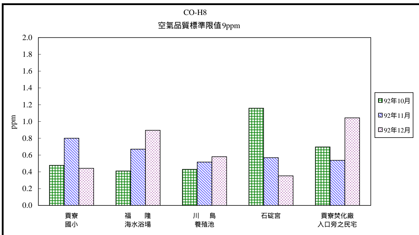
圖2.2-8 核四施工環境監測空氣品質一氧化碳 92年10月至12月最大八小時平均值比較分析圖
