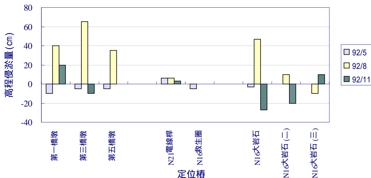
圖 3.1-46 各定位樁相對侵淤量示意圖
