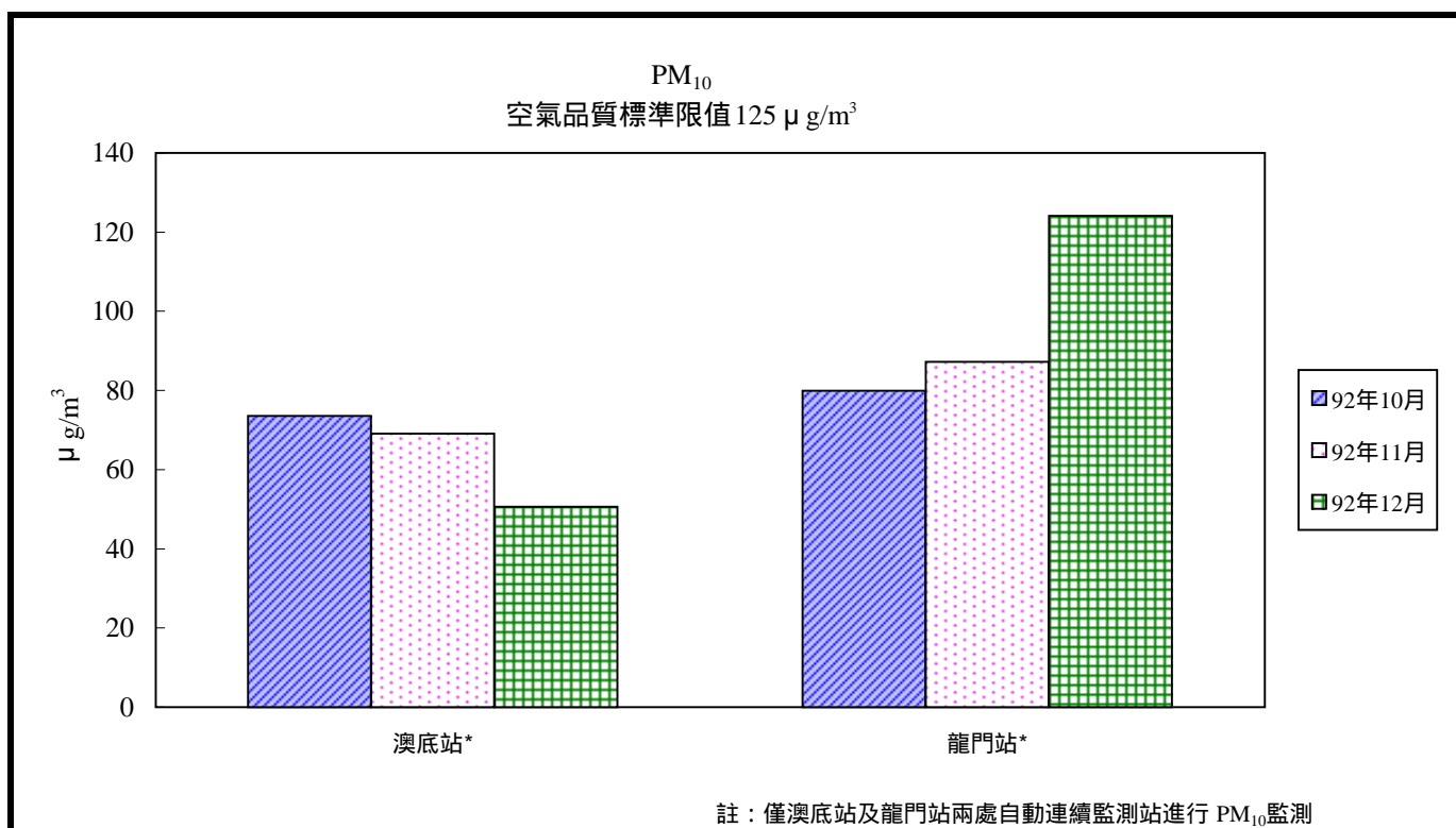
圖2.2-2 核四施工環境監測空氣品質懸浮微粒 92年10月至12月最大日平均值比較分析圖
