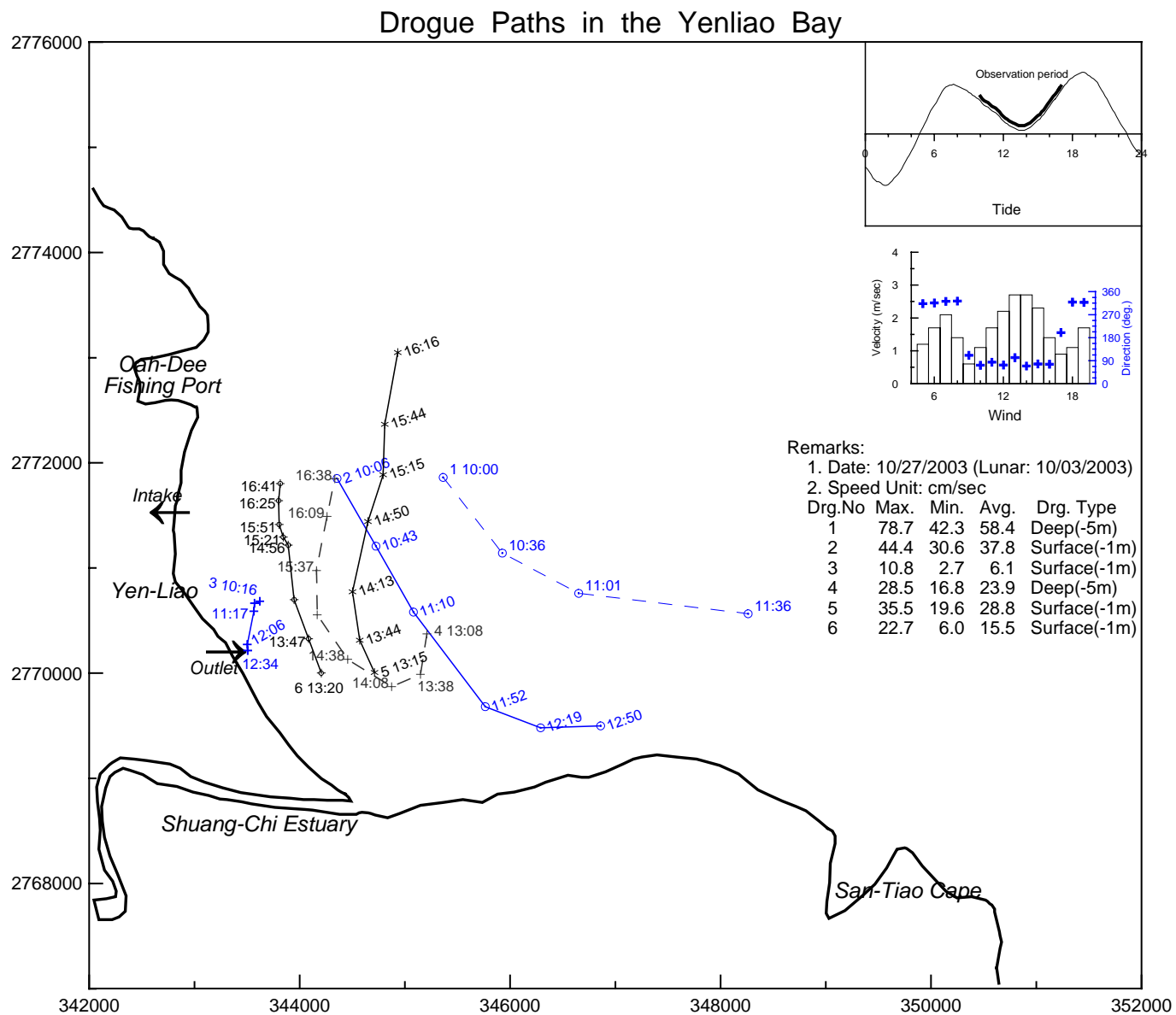
圖2.13-1 核四施工環境監測海象調查92年10月27日漂流浮標追蹤軌跡圖
