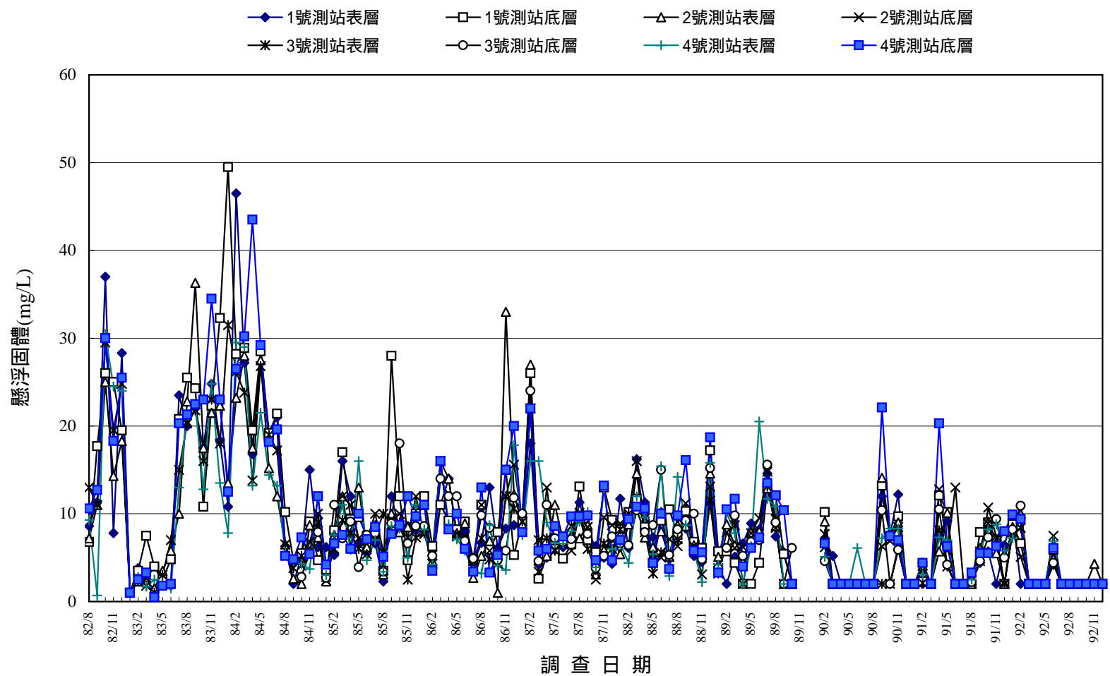
圖3.1-35 核四施工環境監測海域水質歷年調查懸浮固體濃度變化圖
