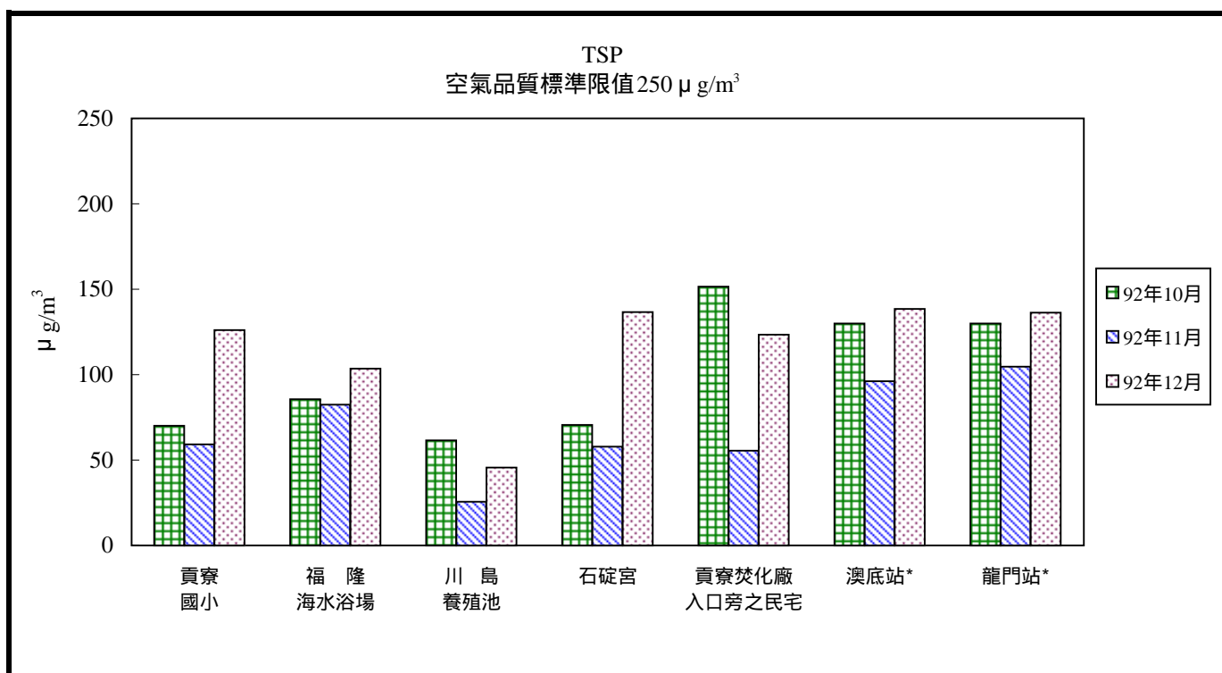
圖2.2-1 核四施工環境監測空氣品質總懸浮微粒 92年10月至12月最大24小時值比較分析圖
