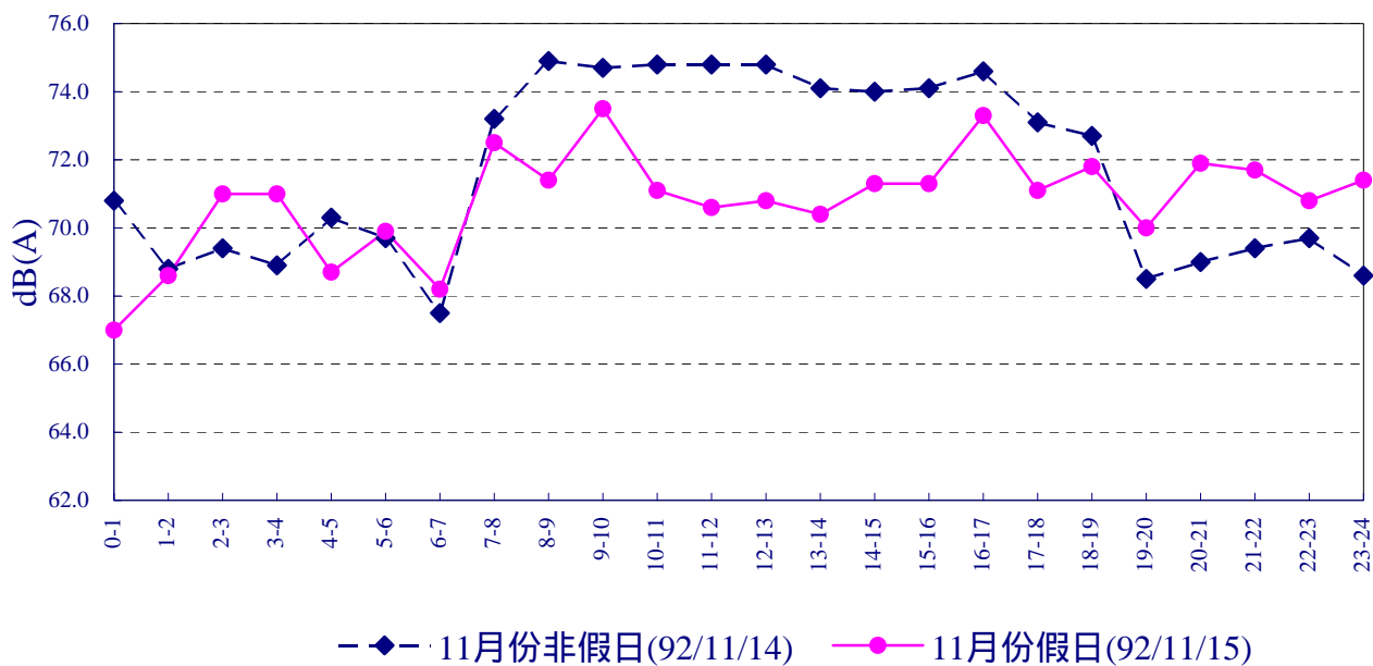
圖2.3-13 核四施工環境監測鹽寮海濱公園 92年11月噪音 L_{eq} 逐時變化圖
