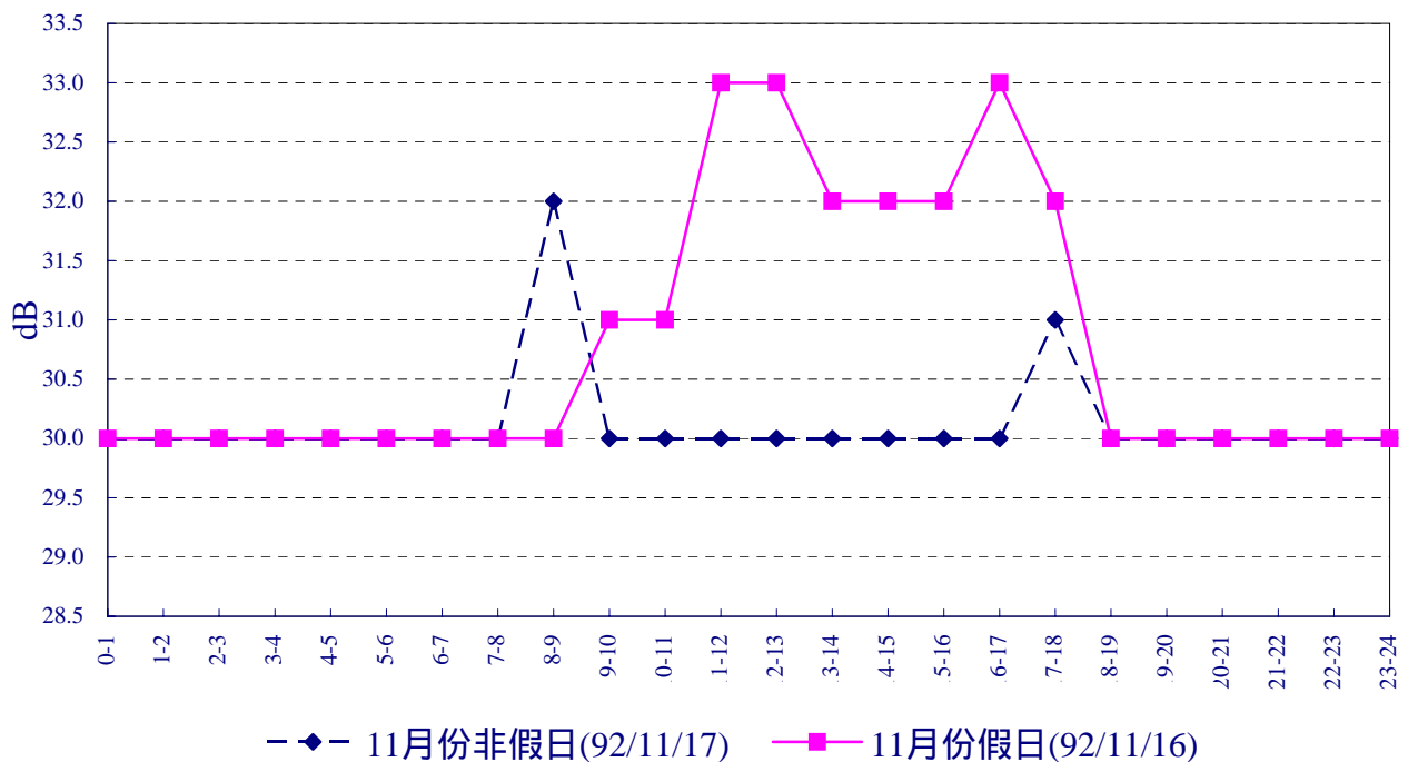
圖2.3-18 核四施工環境監測102縣道之新社橋92年11月振動 L_{v10} 逐時變化圖
