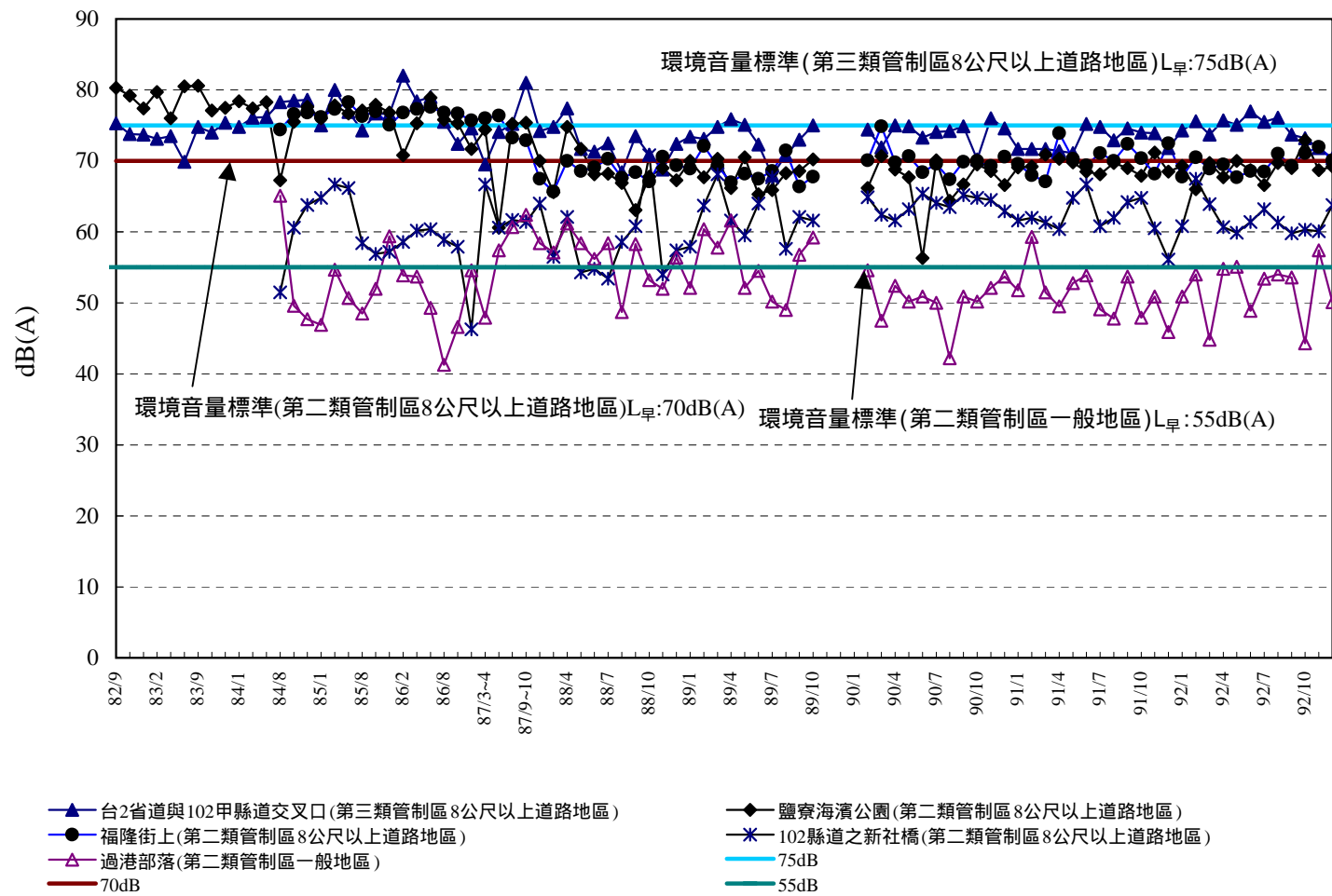
圖3.1-11 核四施工環境監測歷年噪音 L_{\text{早}} 非假日監測結果變化圖
