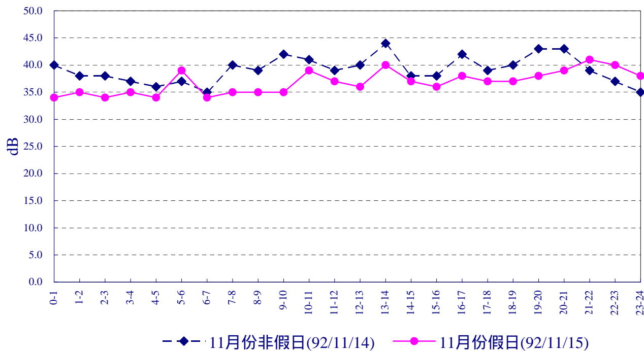
圖2.3-12 核四施工環境監測台2與縣102甲交叉口92年11月振動 L_{v10} 逐時變化圖
