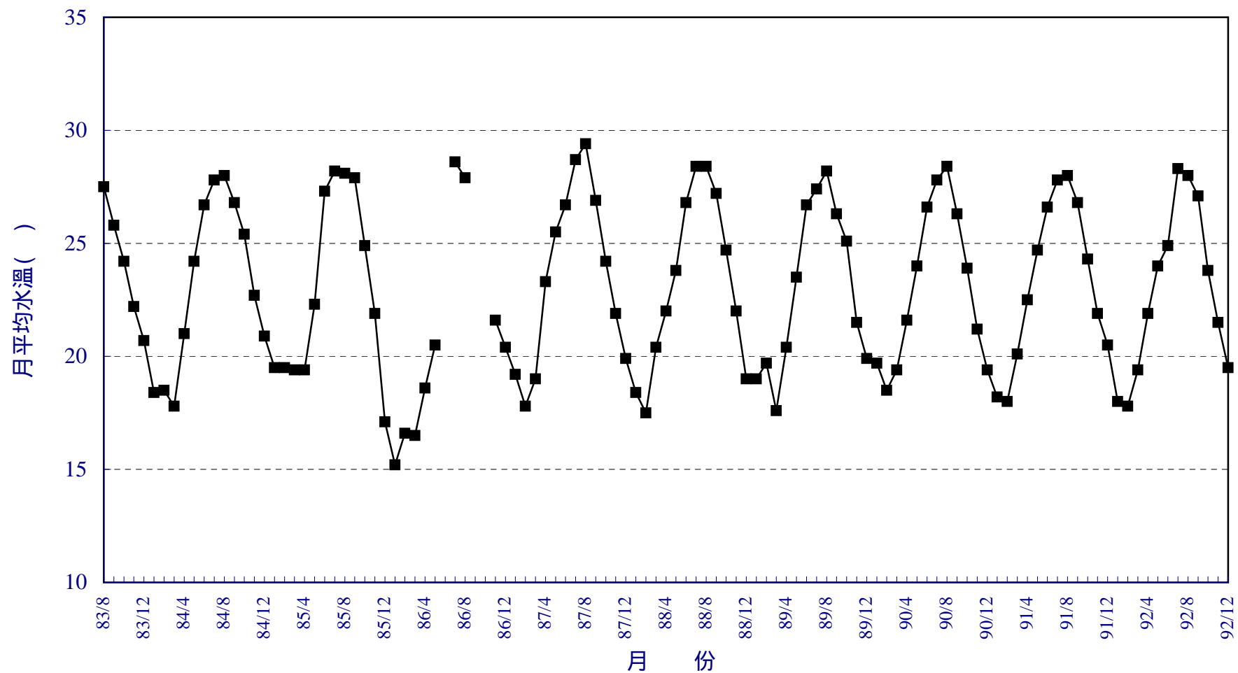
圖 2.13-4 核四施工環境監測海象調查沿岸水溫月平均變化圖 調查日期：83年8月至92年12月
