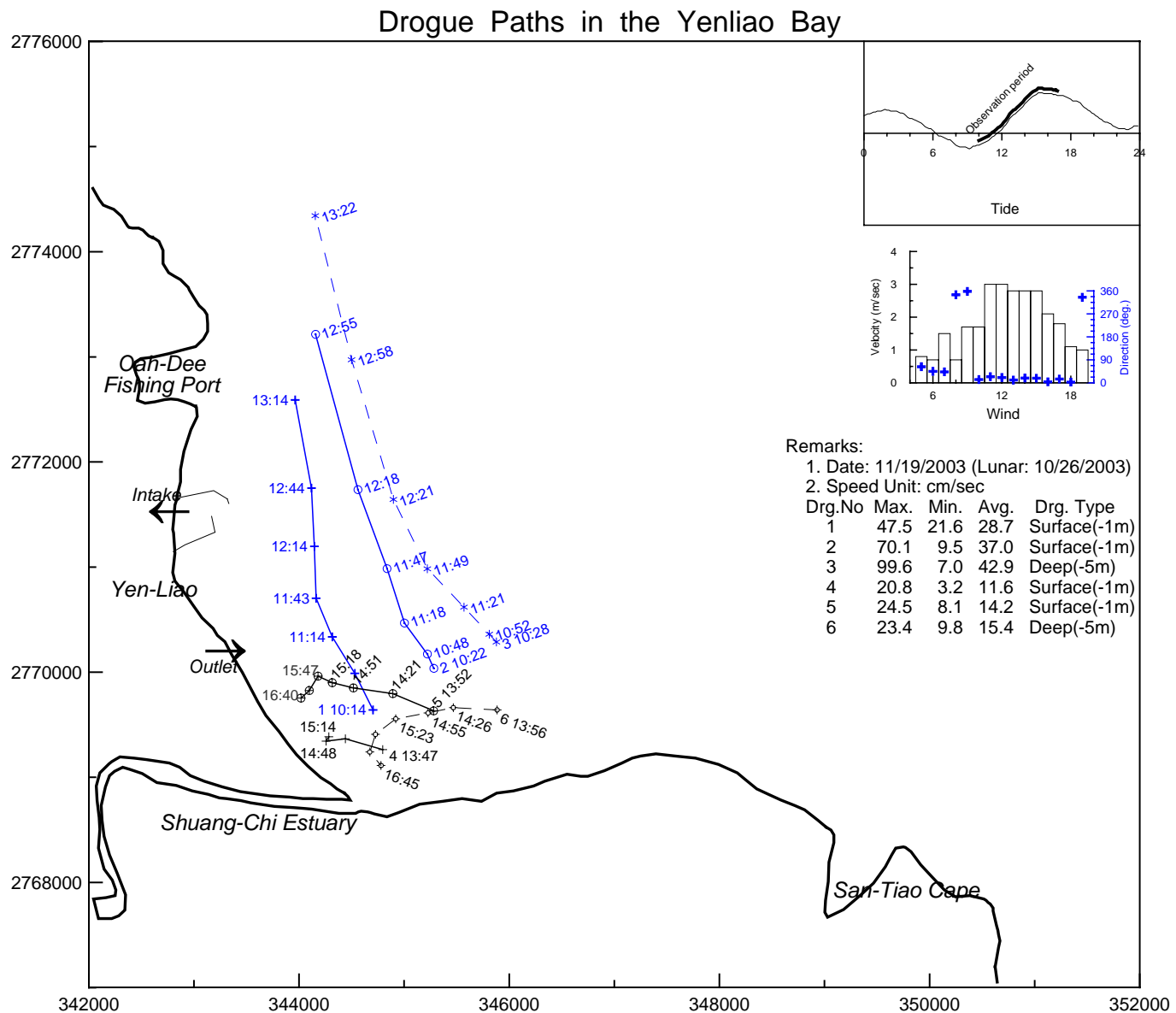
圖2.13-2 核四施工環境監測海象調查92年11月19日漂流浮標追蹤軌跡圖
