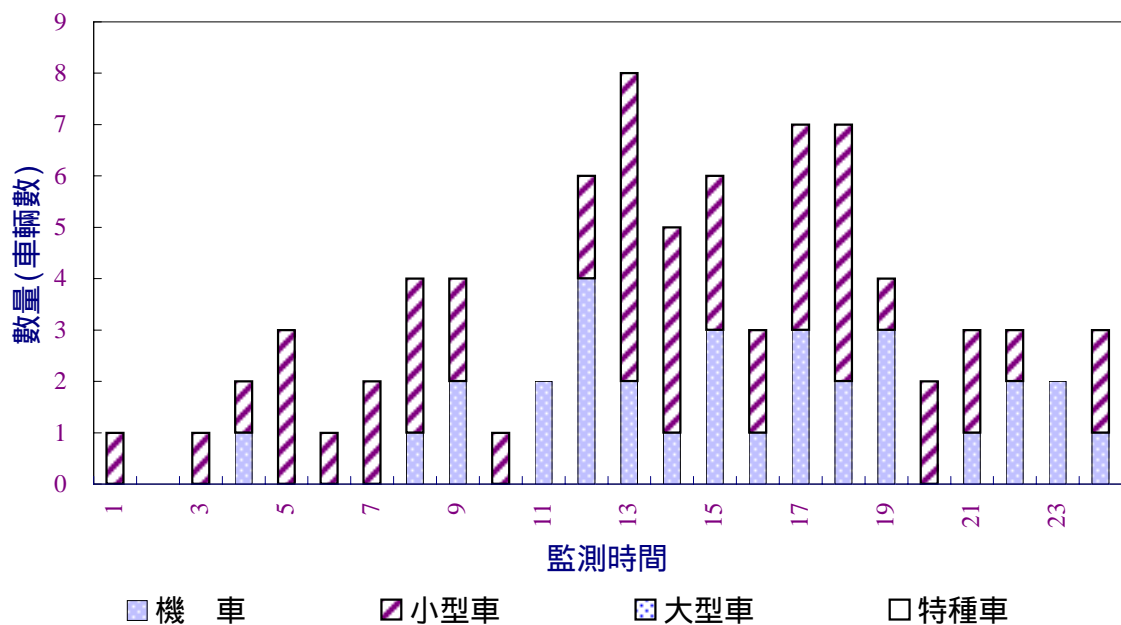
圖2.4-9 核四施工環境監測過港部落 本季非假日(92/10/13)交通量逐時變化圖
