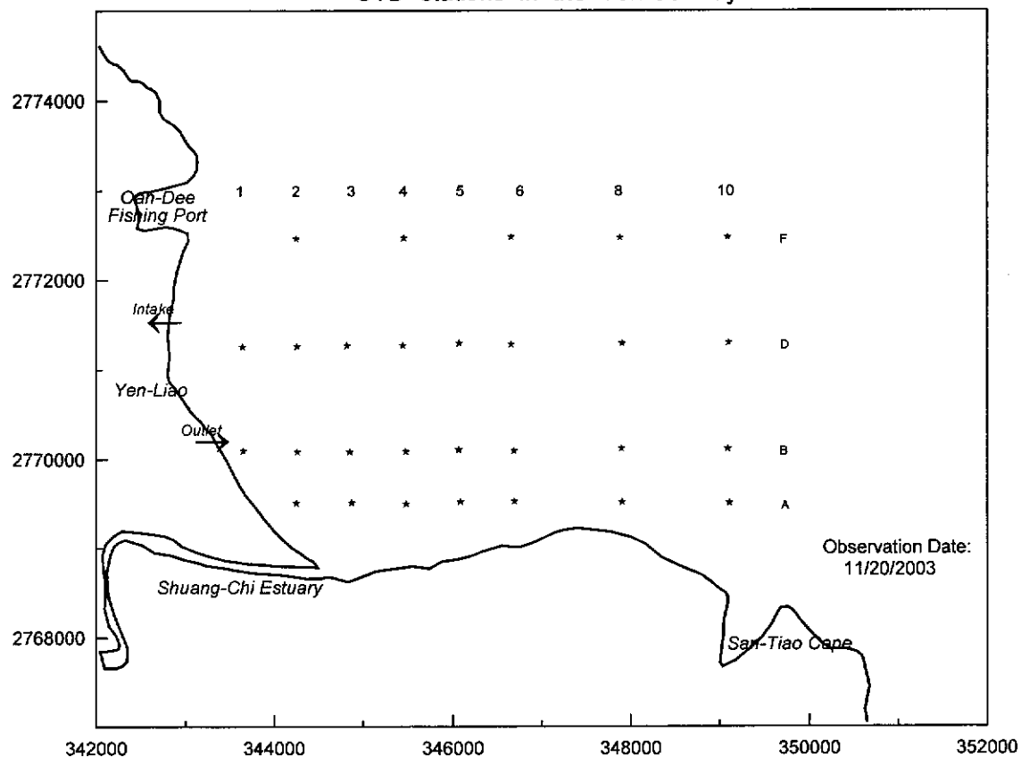
附錄IV.8-2 海象CTD調查92年11月20日縱深剖面溫鹽圖
