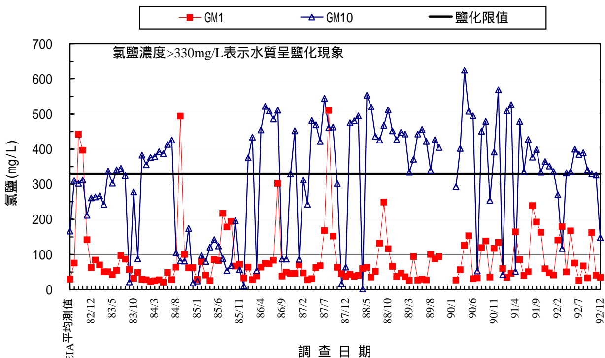
圖3.1-34 核四施工環境監測 GM1及GM10監測井歷年地下水氯鹽監測結果
