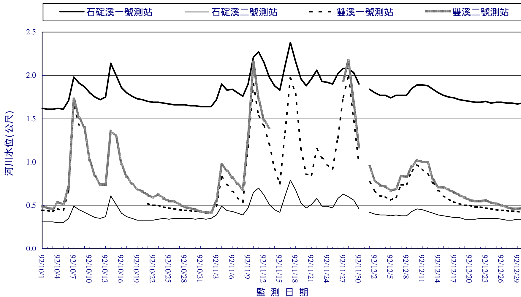
圖2.5-1 核四施工環境監測河川水文 92年10月至12月日平均水位變化圖
