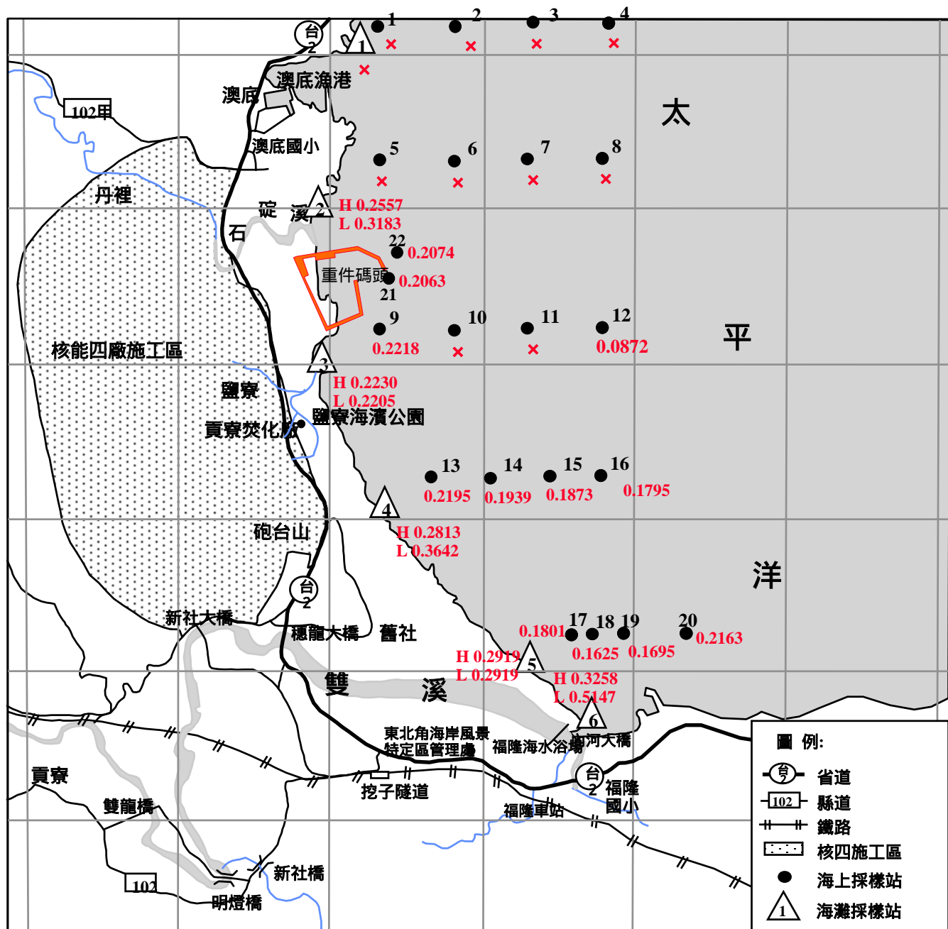
圖2.15-1 核四施工環境監測海域漂砂採樣站累積百分比50%粒徑資料圖(92年11月)
