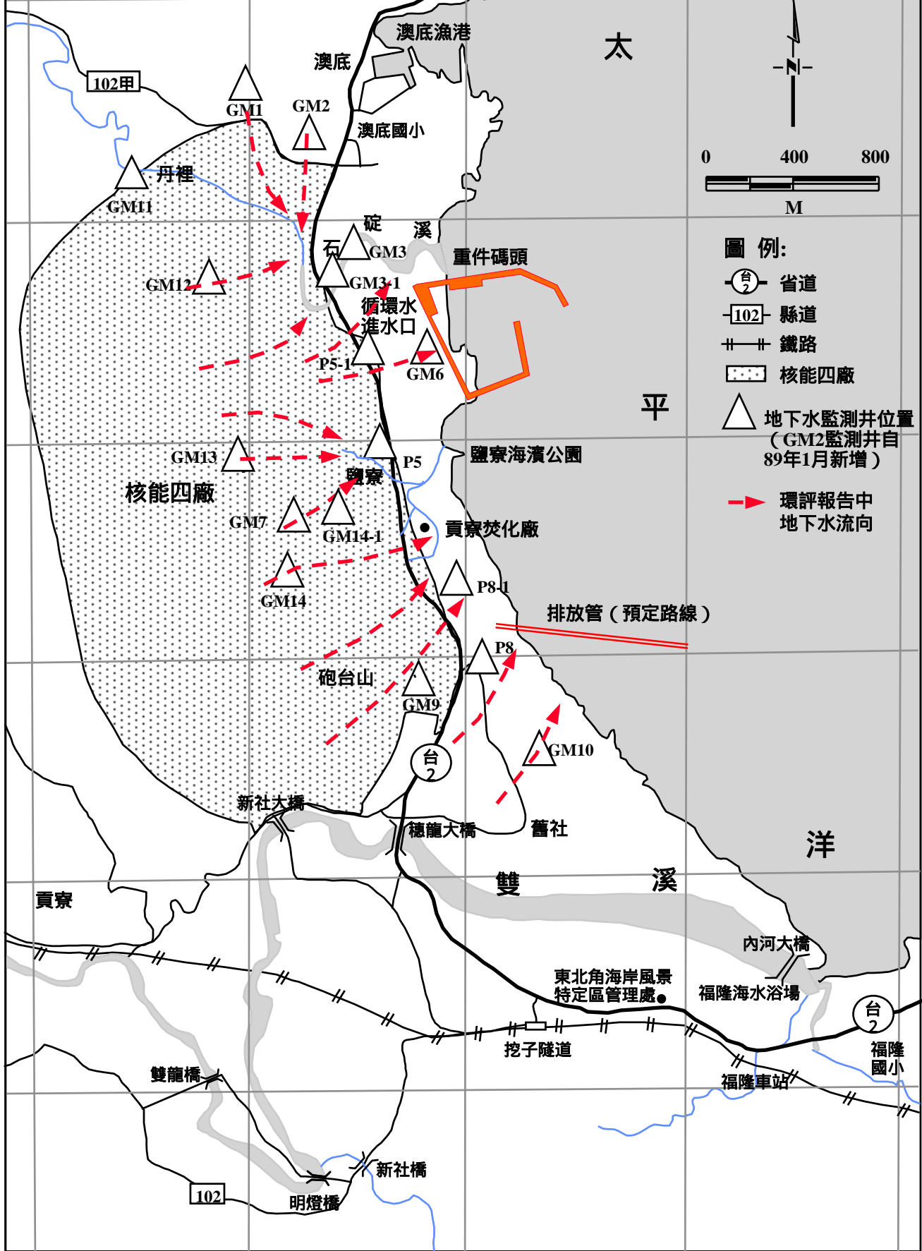
圖2.1.20 核四施工環境監測地下水流向示意圖
