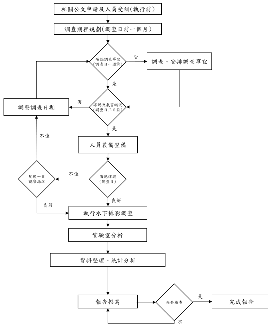
圖 1.6.8-1 水下攝影品保品管流程圖
