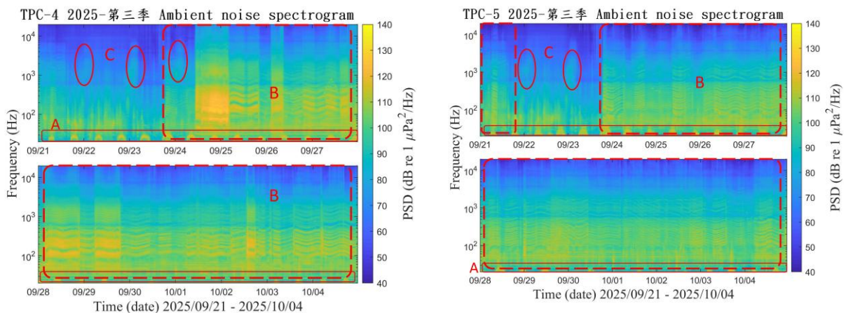
圖 2.8-1 環境噪音時頻譜圖
