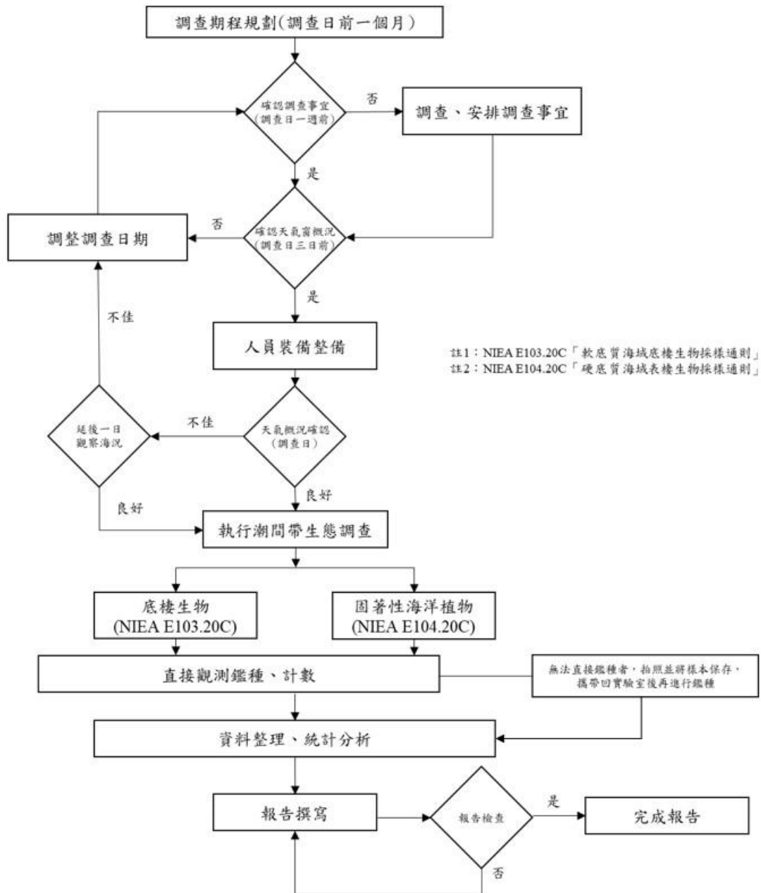
圖 1.6.2-2 海上鳥類生態品保品管流程圖
