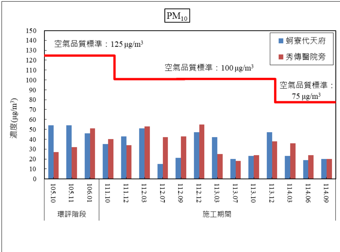
圖 3.1.1-4 歷次懸浮微粒 PM 10 24 小時值變化圖
