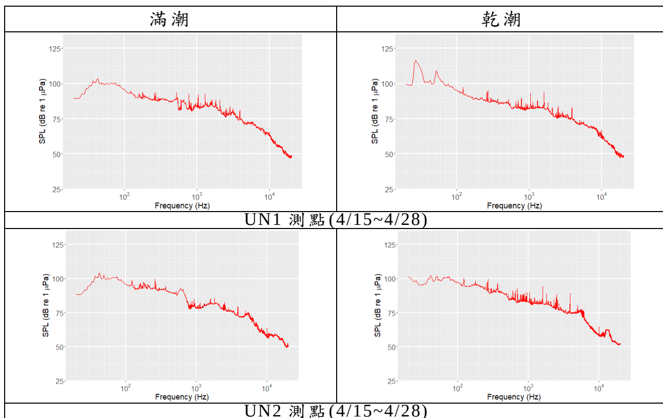
圖 2.7-2 UN1及UN2測點之1 Hz聲壓位準分布
