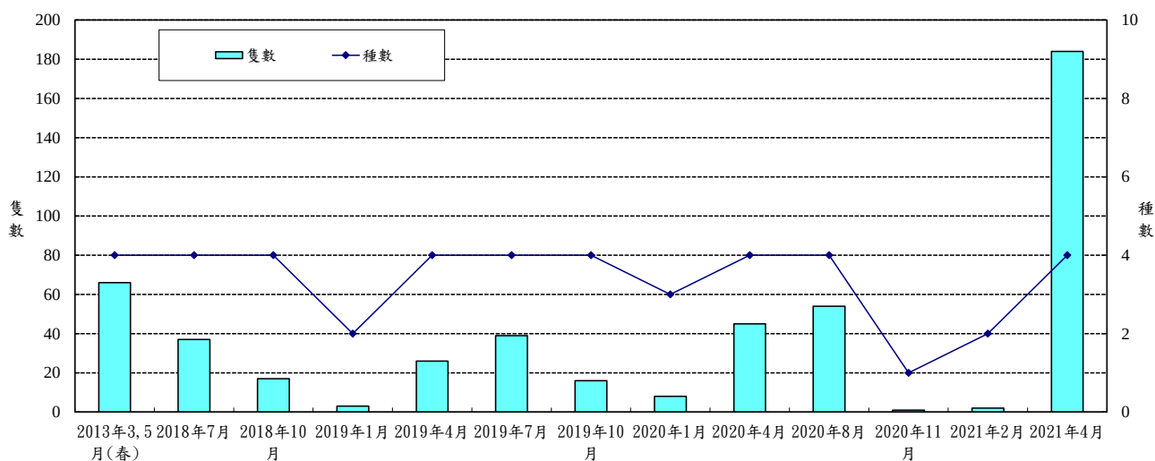
圖3.1-28 兩棲類歷次調查比較圖
