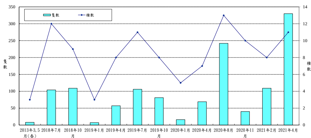
圖3.1-27 哺乳類歷次調查比較圖
