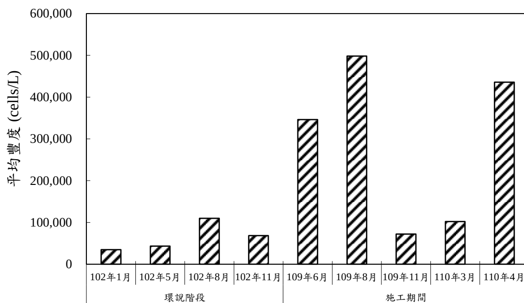
圖 3.1-35 浮游植物生物歷次調查結果趨勢圖
