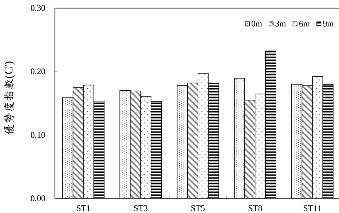
圖 2.6-9 海域各測站浮游動物優勢度變化圖
