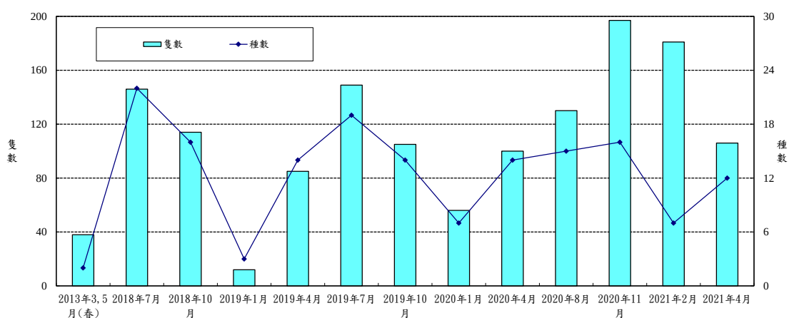
圖 3.1-30 蝴蝶類歷次調查比較圖
