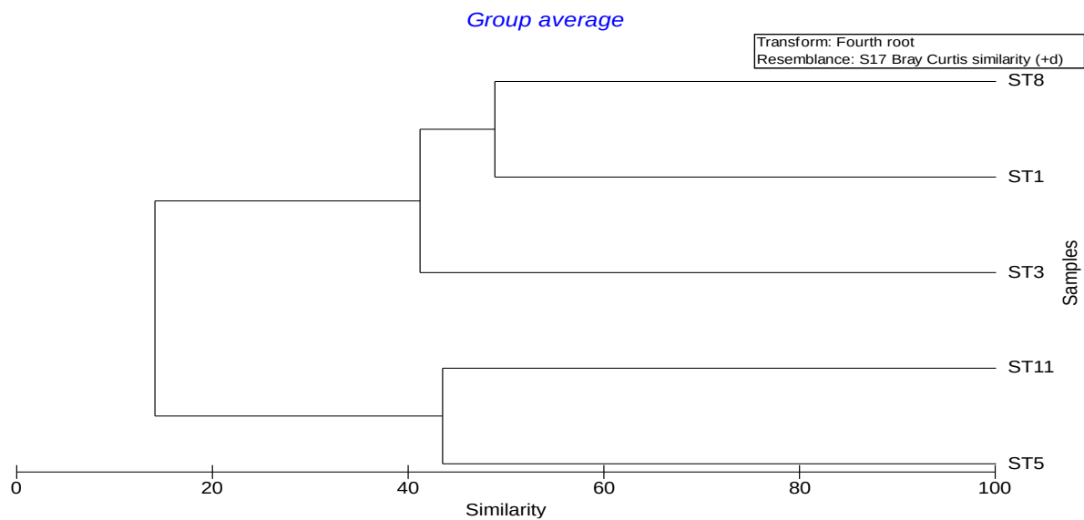
圖 2.6-12 仔稚魚之群集分析樹狀圖
