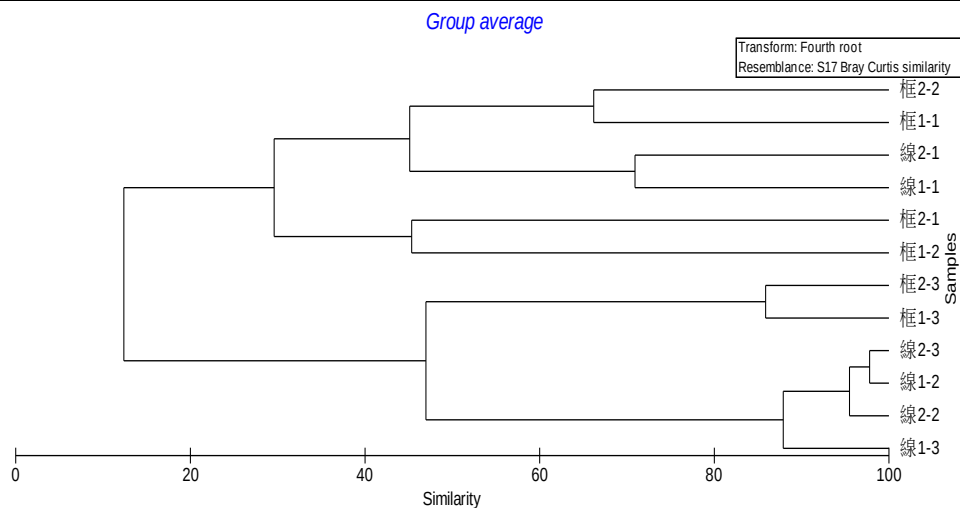
圖 2.6-14 潮間帶底棲生物之各測站群聚分析樹狀圖
