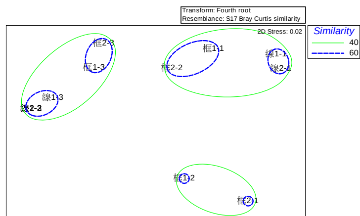
圖 2.6-15 潮間帶底棲生物之各測站群集 MDS 圖
