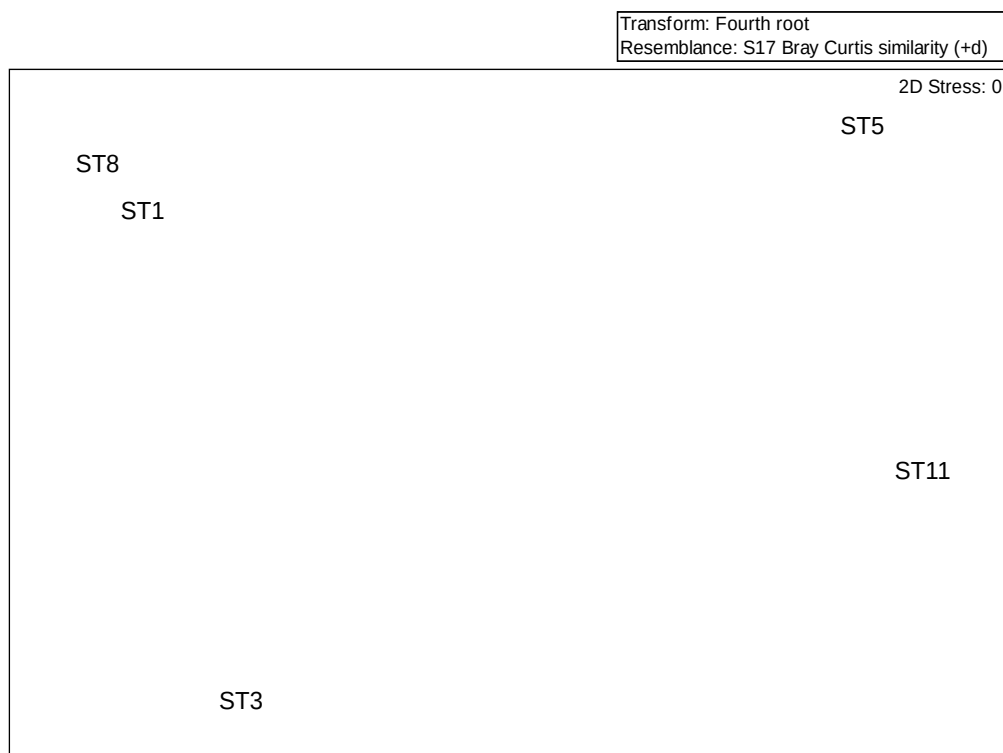
圖 2.6-13 仔稚魚之 MDS 群集分析圖
