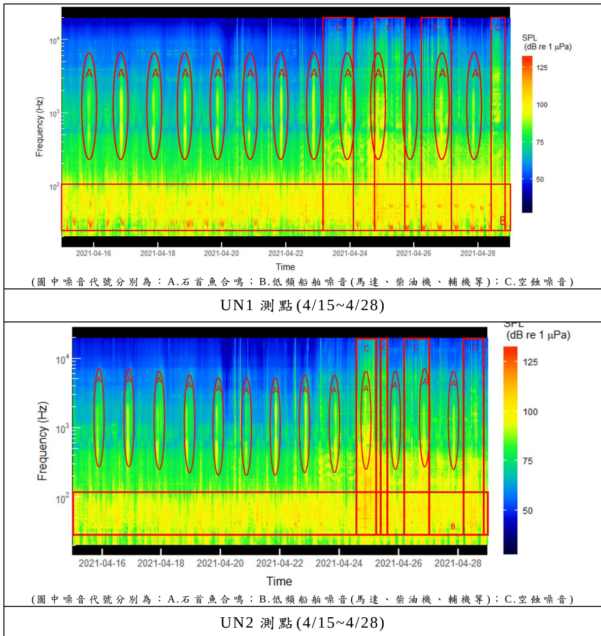
圖2.7-1 UN1及UN2測點時頻譜圖
