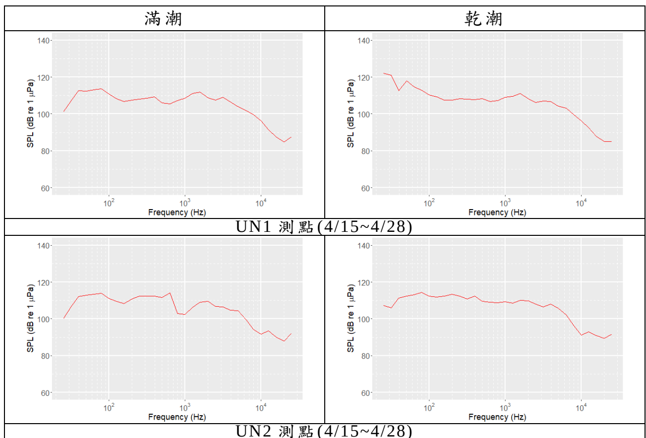
圖 2.7-3 UN1 及 UN2 測點之 1/3 Octave Band 聲壓位準分布
