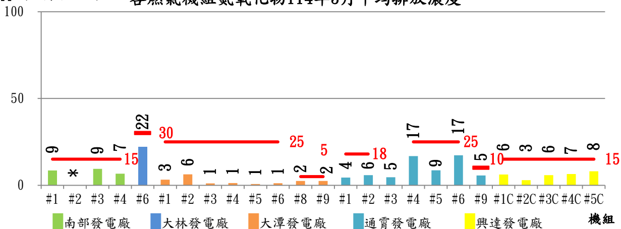
ppm(百萬分之一) 各燃氣機組氮氧化物114年3月平均排放濃度
