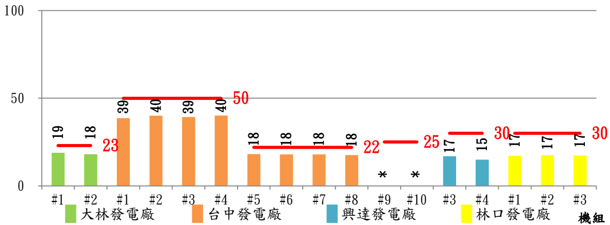
各燃煤機組粒狀污染物114年5月平均排放濃度
